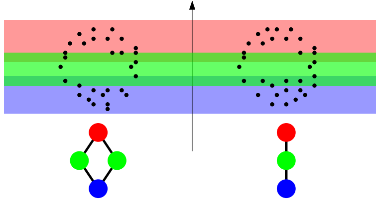
Figure 1.7: Mappers calculés sur des échantillonnages similaires du cercle, avec la fonction hauteur et une couverture composée de trois intervalles.
