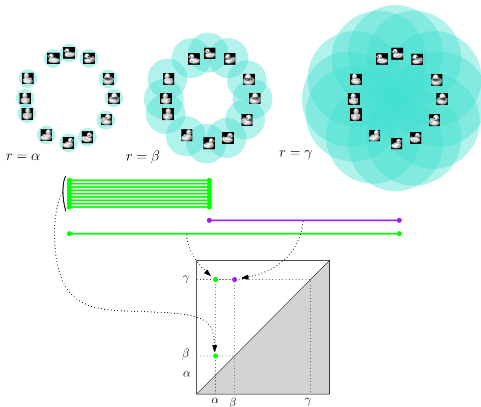
Figure 1.4: Trois différentes unions de boules centrées sur des images vues comme des vecteurs dans un espace Euclidien de grande dimension. L'apparition et la disparition d'attributs topologiques, comme des composantes connexes ou des trous, est enregistrée dans un diagramme de persistance , dans lequel les points représentant des attributs en dimension 0 sont en vert, et ceux représentant des attributs en dimension 1 sont en violet.
