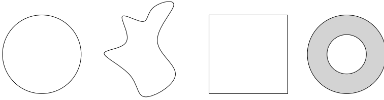
Figure 1.1: Déformations du cercle.
