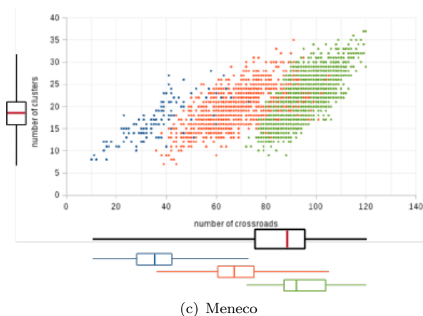
FIGURE 6.8 – Métabolites ME-persistence et clusters des 10 800 réseaux obtenus après complétion de 3600 réseaux dégradés. Chacun des 3 600 réseaux métaboliques dégradés de iJR904 est complété avec trois méthodes de complétion dans l'optique de restaurer la production d'une biomasse correspondante. Les nombres de métabolites ME-persistence et de clusters obtenus pour chacune des méthodes sont représentés dans les sous-figures correspondantes. Les différentes couleurs correspondant à la classification des réactions de biomasse donnée dans la Figure 6.6.
