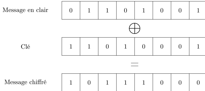
FIGURE 5.1 – Communication chiffrée par une méthode XOR
