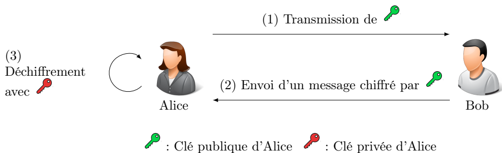
FIGURE 5.2 – Envoi d'un message par chiffrement asymétrique
