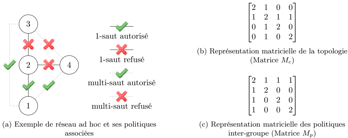
FIGURE 6.1 – Utilisation des matrices M_c et M_p pour la représentation de communications et de politiques ad hoc inter-groupe
