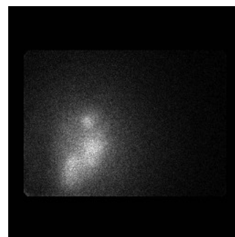
(b) ^{90}\text{Y} bremsstrahlung SPECT
