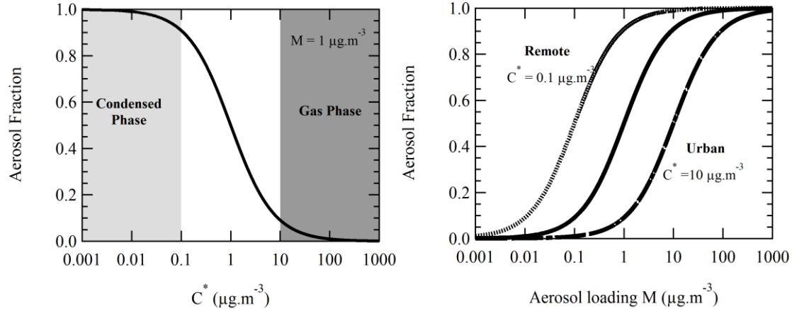
FIGURE 1.9 – Partitionnement entre la phase gazeuse et la phase particulaire selon la concentration saturante C^* avec M = 1 \mu\text{g}\cdot\text{m}^{-3} (gauche). Illustration de ce partitionnement pour des atmosphères plus ou moins polluées ( M = 0.1, 1, 10 \mu\text{g}\cdot\text{m}^{-3} ) (droite).
