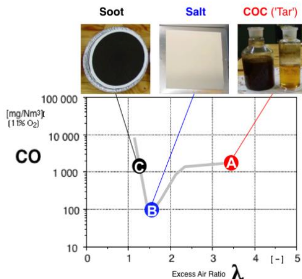
FIGURE 1.31 – Caractéristique de l'aérosol organique selon les conditions de combustion. COC se réfère à Condensable Organic Compounds , et soot à un aérosol riche en carbone élémentaire. Au point A la température de combustion est abaissée. Aux points B et C, elle est élevée (Nussbaumer et al., 2010).
