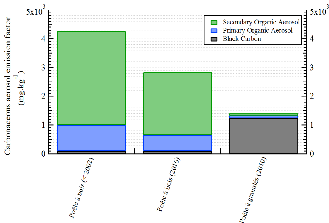
FIGURE 3.1 – Facteurs d’émission moyens de la fraction carbonée de l’aérosol émis par des appareils pour le chauffage au bois résidentiel et leur potentiel de formation d’aérosol secondaire après une exposition à OH de 5 \times 10^6 molécules.cm -3 .h. Poêle à bois (<2002) : 5 étoiles Flamme Verte, Poêle à bois (2010) : 7 étoiles Flamme Verte, Poêle à granulés : 5 étoiles Flamme Verte.
