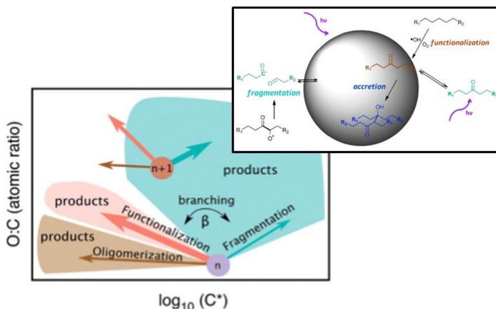
FIGURE 1.14 – Effet des différents mécanismes de vieillissement des émissions – fonctionnalisation, oligomérisation ou accréation, fragmentation – sur la volatilité et le degré d’oxydation de l’aérosol organique. D’après Jimenez et al. (2009) et Chacon-Madrid and Donahue (2011).
