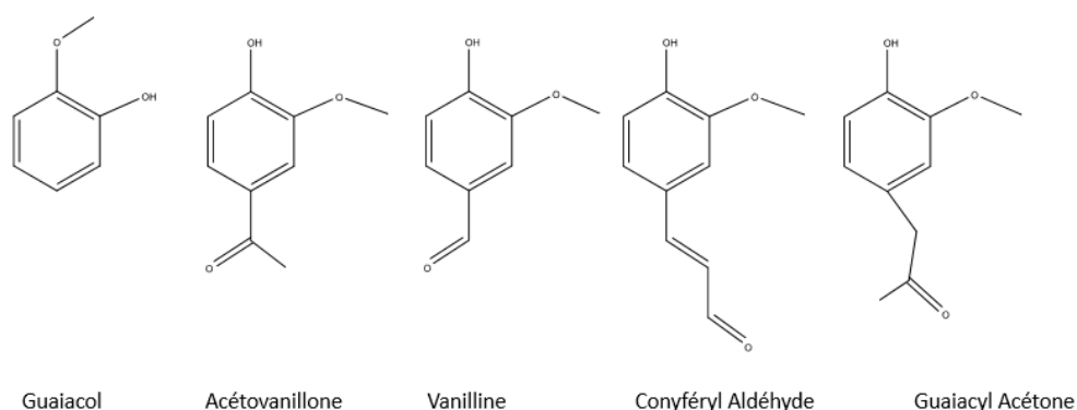
FIGURE 1.34 – Structures chimiques des composés dérivés du guaïacol et issus de la dégradation du conyféryl alcool.
