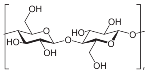
FIGURE 1.29 – Structure de la cellulose composés du monomère D-glucose.
