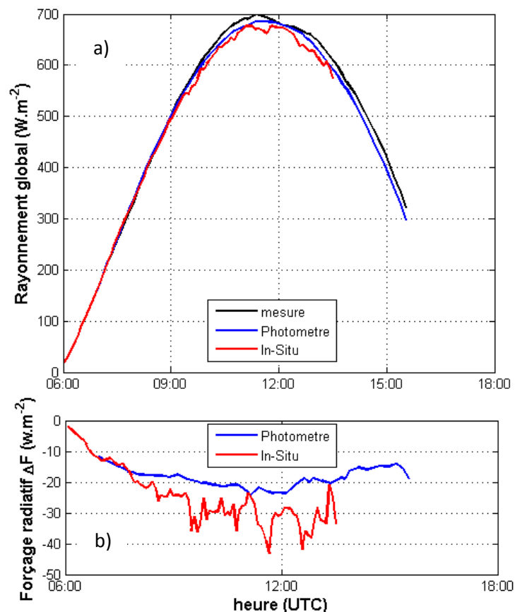
Figure 5.12 : a) Rayonnement global de surface mesuré par un pyranomètre en noir et établi à partir du modèle SBDART et des mesures photométriques (en bleu) ou des mesures in-situ (en rouge). b) forçage radiatif issu des deux méthodes pour la journée du 30 Septembre 2015.
