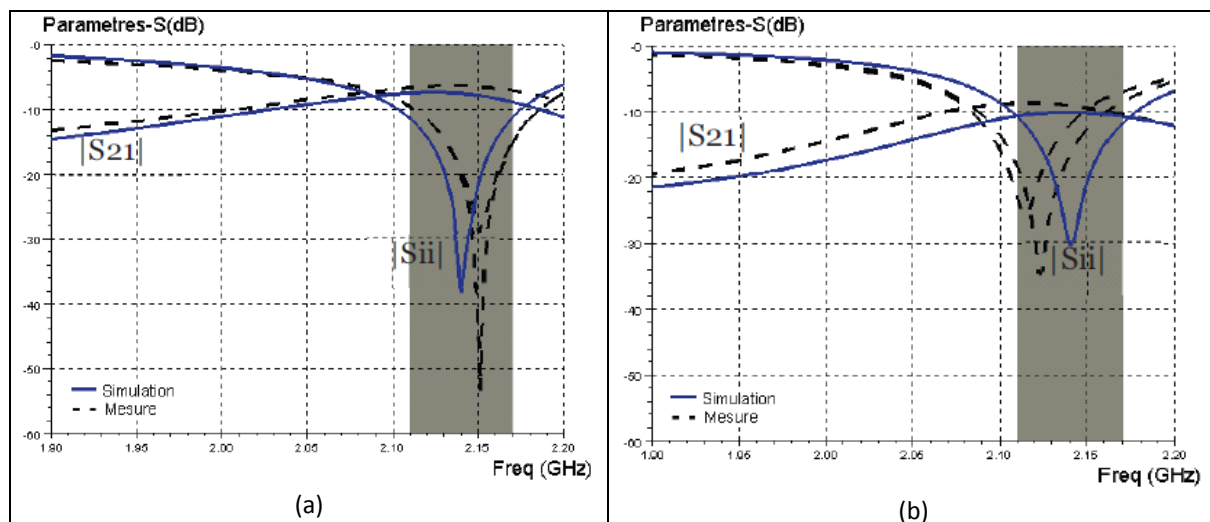
Figure 32: Paramètres S simulés et mesurés des systèmes sans (a) et avec (b) lignes verticales extérieures repliées
