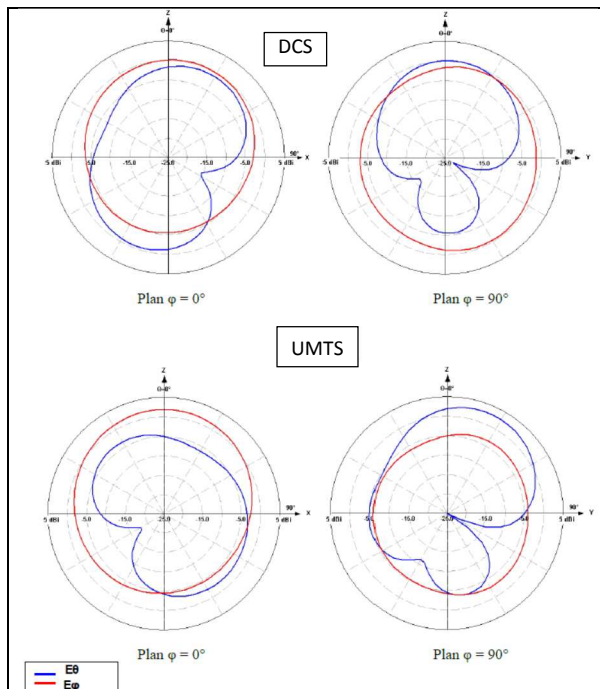
Figure 9: Diagrammes de rayonnement en gain des antennes PIFAs DCS/UMTS associées sur un même PCB quand les languettes de courts-circuits se font face et sans ligne de neutralisation
