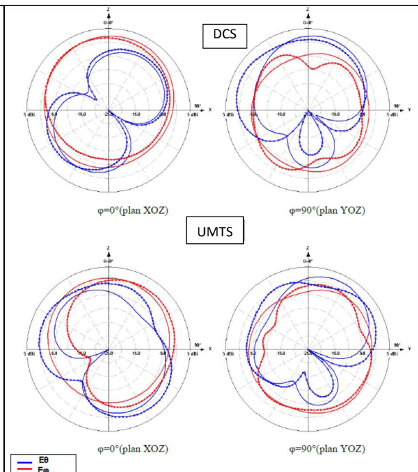
Figure 10: Diagrammes de rayonnement en gain simulés (ligne continue) et mesurés (ligne avec croix) des antennes PIFAs DCS/UMTS associées sur un même PCB quand les languettes de courts-circuits se font face et reliées par la ligne de neutralisation
