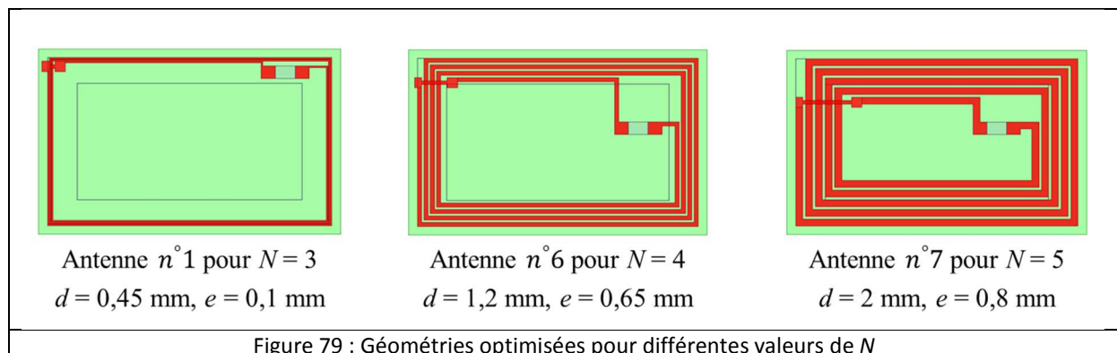
Figure 79 : Géométries optimisées pour différentes valeurs de N
