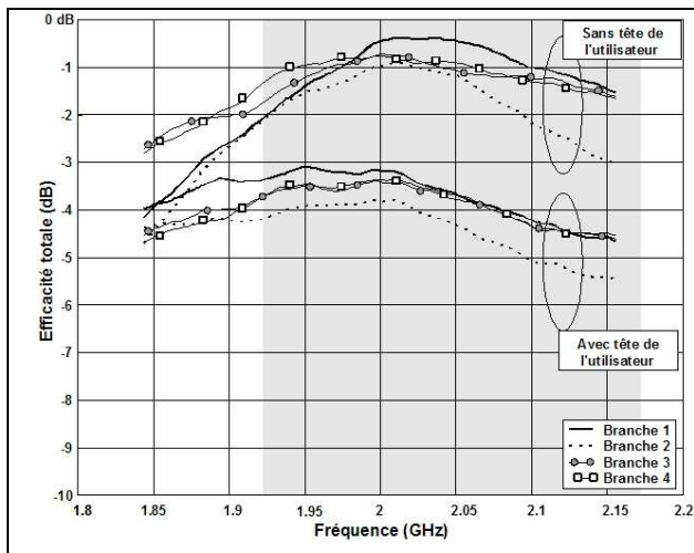
Figure 19: Efficacités totales mesurées en chambre réverbérante à 2 GHz d'un système à quatre antennes « neutralisé » avec et sans la tête de fantôme
