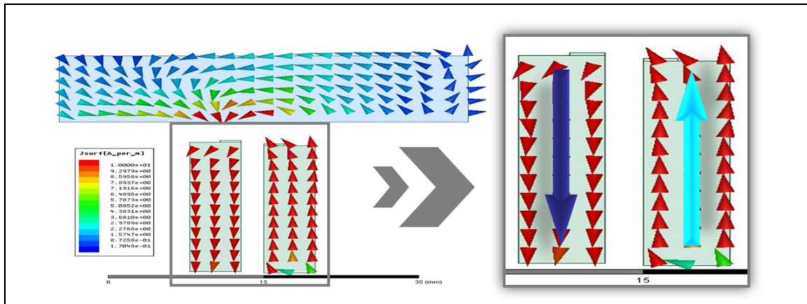
Figure 165 : Densité des courants à la surface des éléments rayonnants de la structure tri-bande initiale
