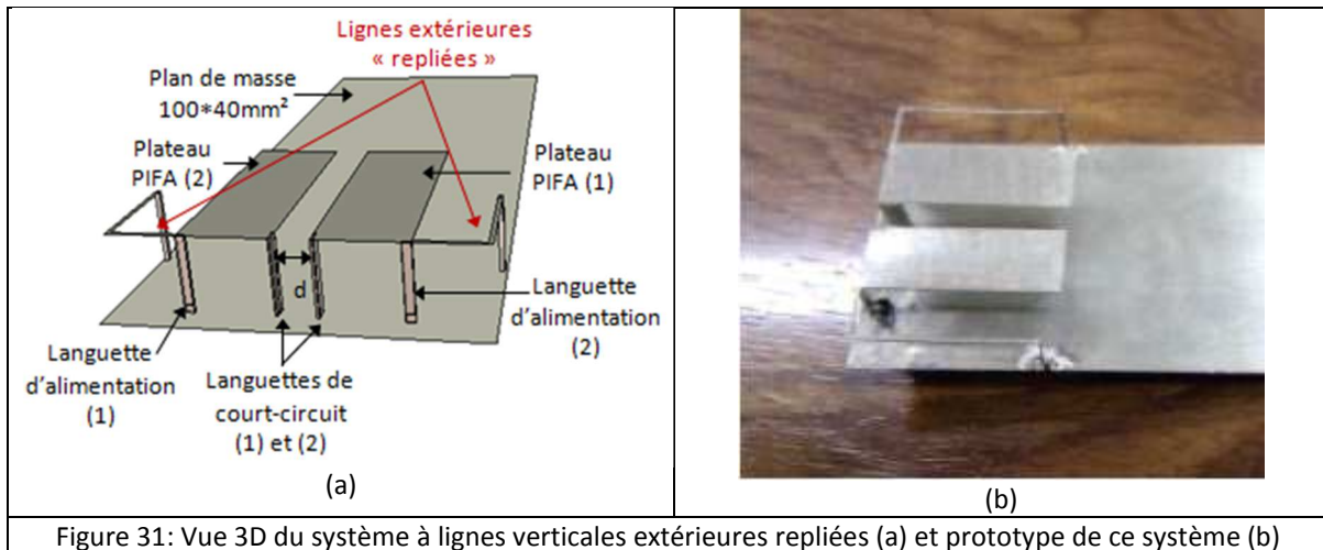
Figure 31: Vue 3D du système à lignes verticales extérieures repliées (a) et prototype de ce système (b)
