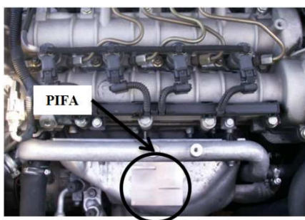
Figure 146 : PIFA avec capteur placée sur le cache collecteur d'un moteur de voiture
