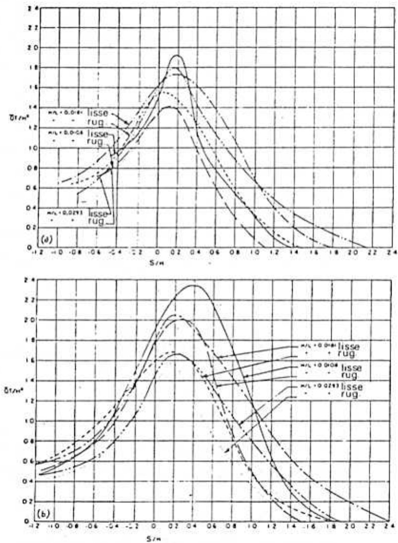
FIGURE 38 FRANCHISSEMENT DES STRUCTURES EN PENTE, PAR RAPPORT A LA CAMBRURE DE LA HOULE INCIDENTE h = 1.69 \text{ ft} , T = 1.25 \text{ sec} , \lambda = 7.17 \text{ ft} , h/\lambda = 0.236 , (a) 1/2 , (b) 1/3
