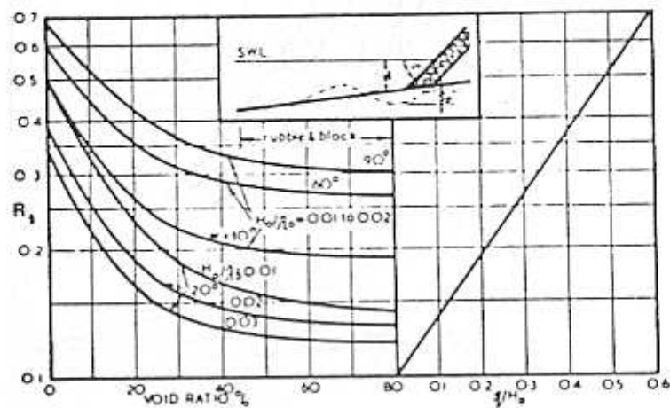
FIGURE 13 INFLUENCE DE LA POROSITE SUR LE COEFFICIENT DE REFLEXION, ET SOUBASSEMENTS s_1 , DUS A LA REFLEXION DE LA HOULE (d'après SAWARAGI 1966 et STRAUB 1957)
