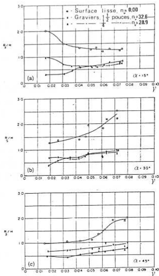
FIG. 24 - HAUTEUR D'ASCENSION RELATIVE R_s/H , PAR RAPPORT A LA CAMBRURE ET LA POROSITE DE LA STRUCTURE POUR ANGLES DE PENTE 15^\circ, 30^\circ, 45^\circ AVEC h/\lambda = 0.218 (d'après K.N. GRANTHEM)
