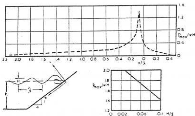
FIGURE 116 - Pressions dues à la houle déferlante sur des structures en plan incliné (pente de 1/4, d'après SKLADNEV et POPOV).
