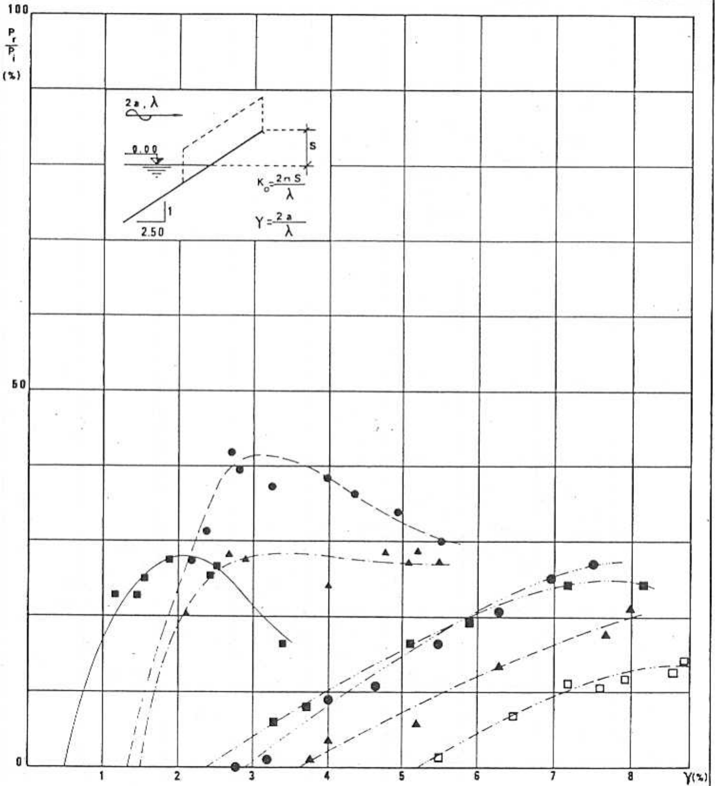
TRIEDRES A HOULE Rapport P_r/P_i (flux d' énergie récupéré/flux d' énergie incident) et cambrure de la houle \gamma pour r=3.75 r = \frac{\text{ouverture avant du trièdre}}{\text{ouverture arrière du trièdre}} K_0=0.100 K_0=0.200 K_0=0.300 K_0=0.400 K_0=0.500 K_0=0.600 K_0=0.700 ■ ● ▲ ■ ● ▲ □
