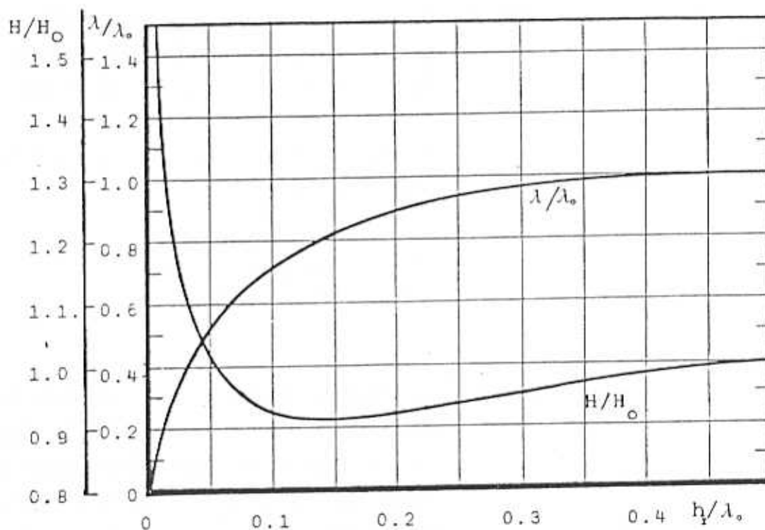
Fig. 3 - Transformations de \lambda et H par rapport à la profondeur h_1
