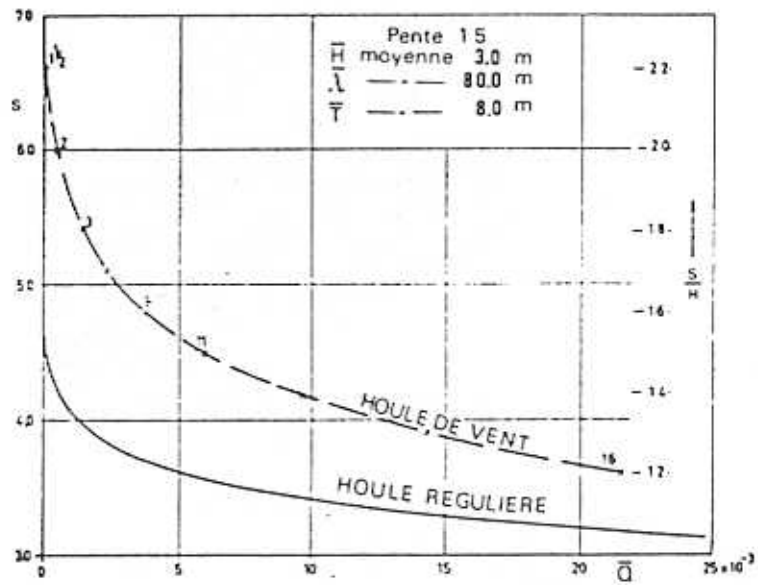
FIGURE 42 FRANCHISSEMENT EN HOULE DE VENT ET REGULIERE. LES NOMBRES INDIQUENT LE POURCENTAGE DES VAGUES QUI FRANCHISSENT LE SEUIL (d'après A. PAAPE)
