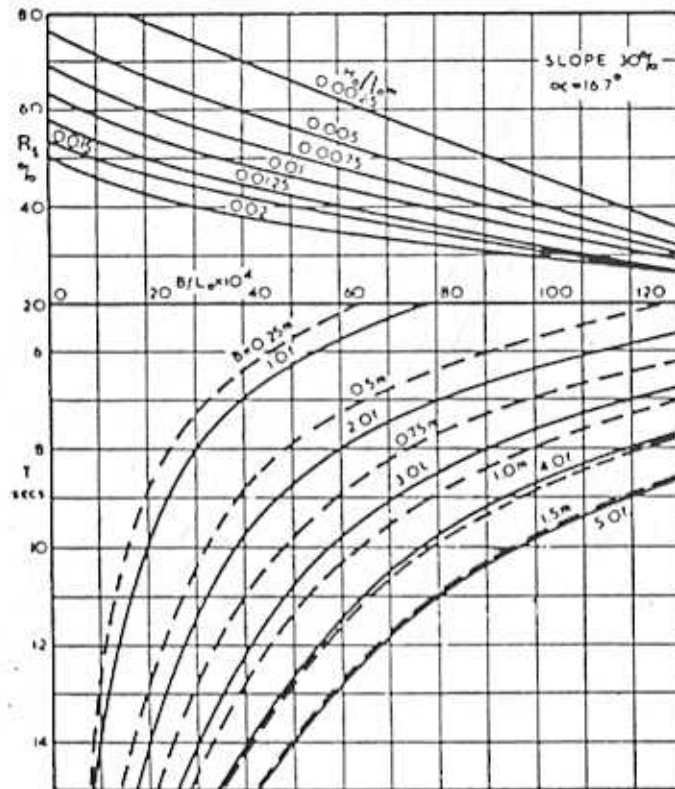
FIGURE 12 INFLUENCE DE LA RUGOSITE SUR LE COEFFICIENT DE REFLEXION POUR UNE PENTE DE 30 % (d'après MORAES 1970)
