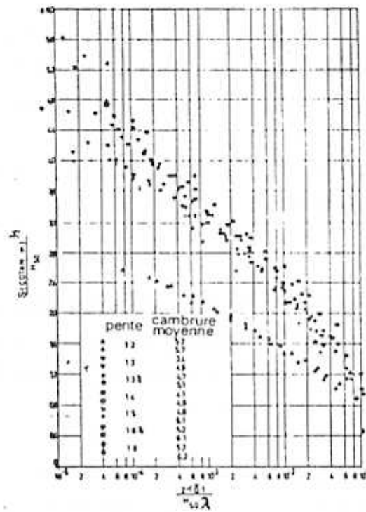
FIGURE 41 LE FRANCHISSEMENT COMME FONCTION DE \frac{h(\cot \alpha \lambda)}{H_{50}} H_{50} = L'AMPLITUDE QUI EST DEPASSEE PAR LE 50 % DES HOULES D'UN ENREGISTREMENT (d'après A. PAAPE)
