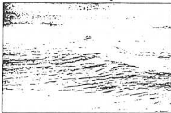
Spilling breaker
