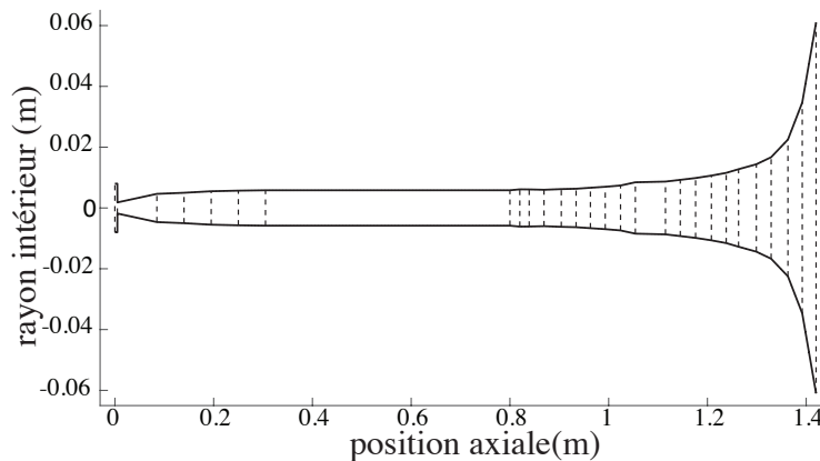
Figure 2.10 Discretisation de la perce R(x) par des tronçons de cônes et de cylindres.
