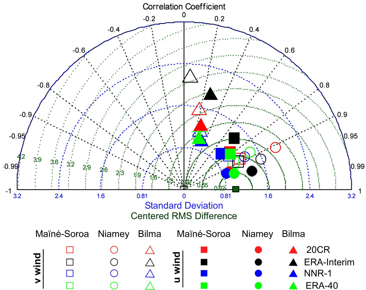
Figure 38 : Comparaisons des séries mensuelles u et v des vents observés et des réanalyses à 10 m du sol, de 1950 à 2009
