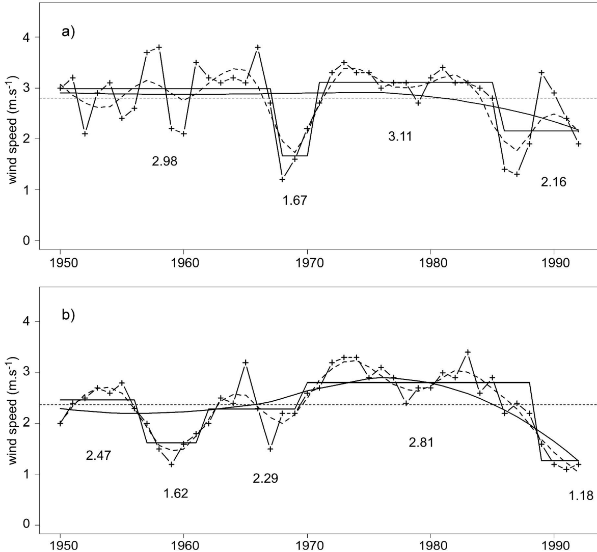
Figure 31 : Vitesses moyennes annuelles (de 6h, 12h et 18h) et tendances à Maïné-Soroa (a) et à Nguigmi (b).
