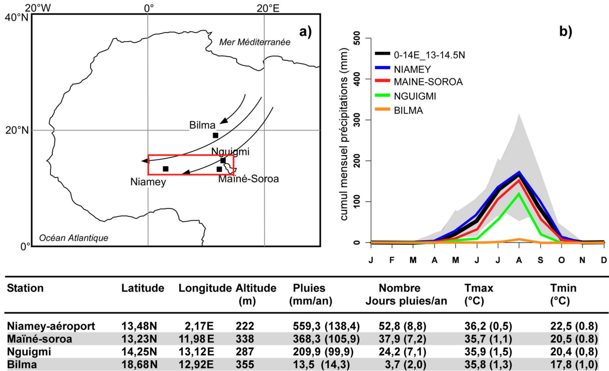
Figure 20 : Localisation des stations, cumuls mensuels des précipitations et quelques traits climatiques.
