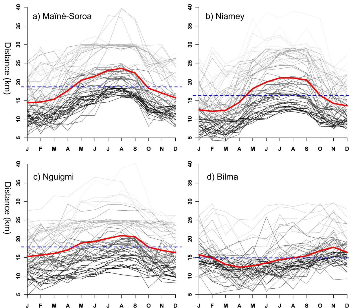
Figure 48 : Régime saisonnier des visibilités horizontales entre 1950 et 2009.
