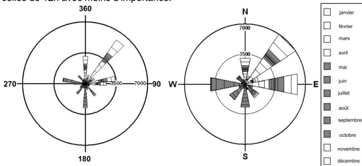
Figure 2 : Nombre d'observations journalières (6h, 12h et 18h) de directions cumulées pour la période 1950-1992 (a= directions en dizaine de degrés et b= directions en secteurs de 22.3 °)
