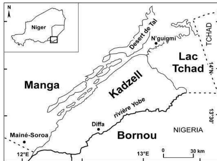
Figure 1 : Localisation et domaines géomorphologiques
