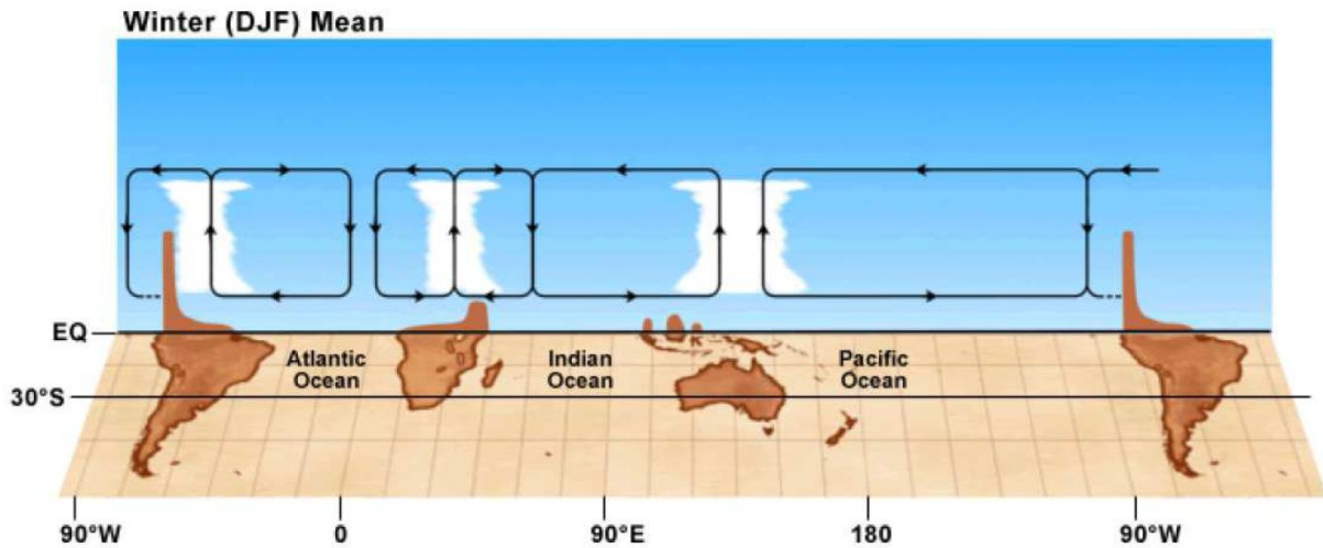
Figure 4 : Circulation de Walker moyenne en hiver entre décembre et février (DJF) ( http://www.meted.ucar.edu ).
