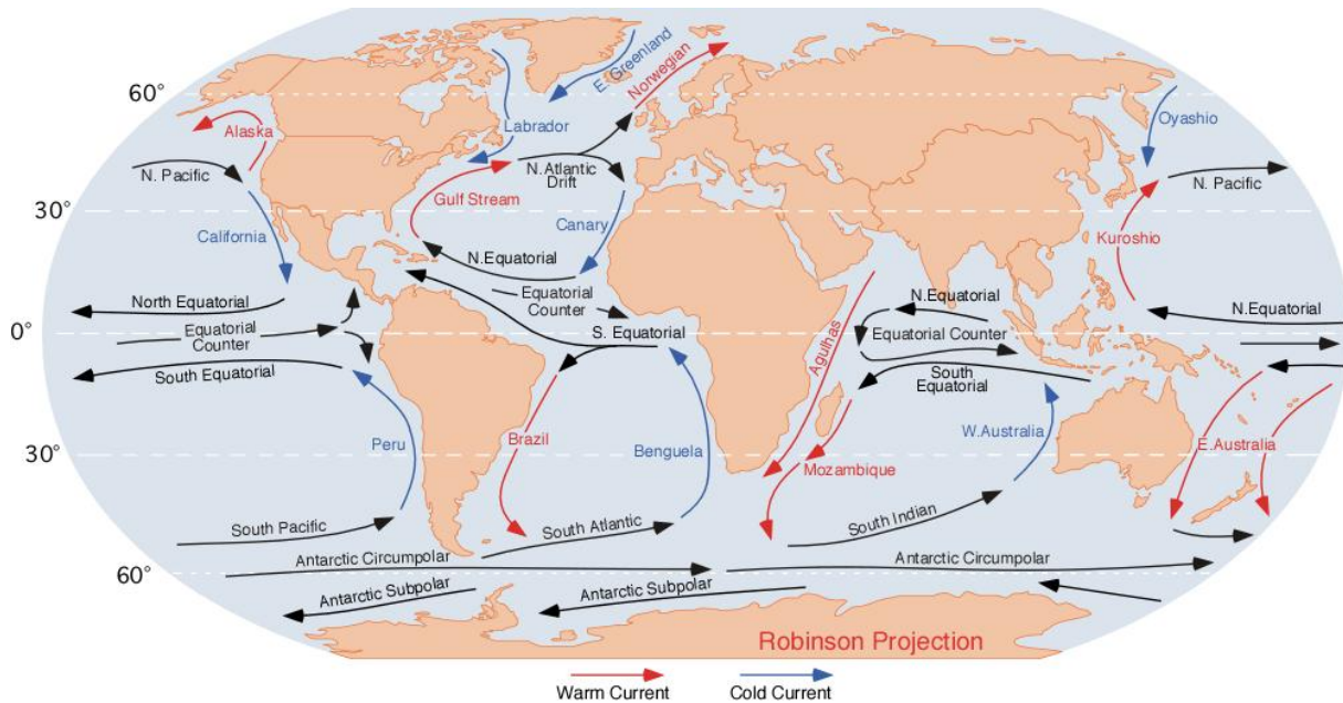
Figure 5 : Les courants marins de surface (www.physicalgeography.net).
