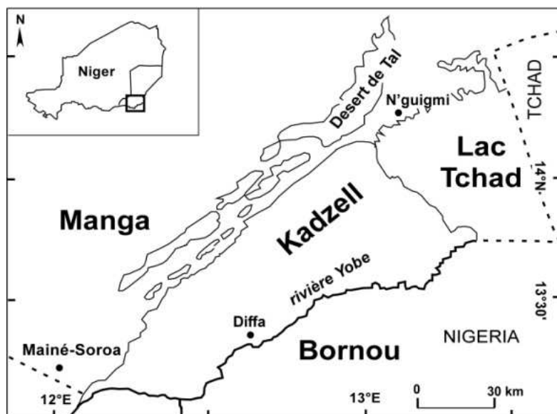
Figure 1 : Localisation et domaines géomorphologiques
