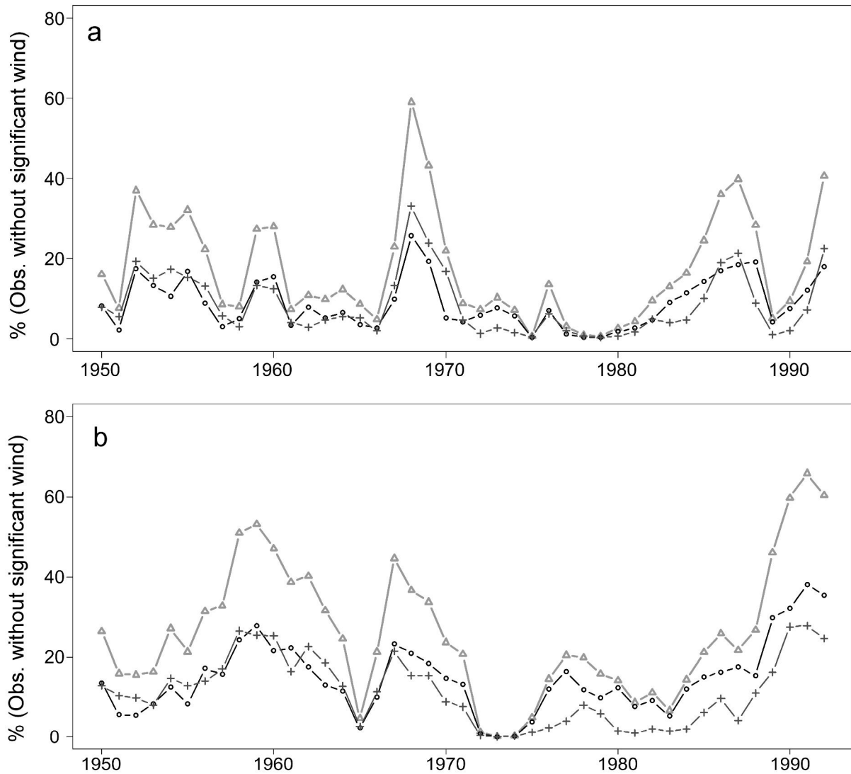
Figure 35 : Pourcentage des observations sans vent significatif pour le total des mesures à 6h 12h et 18h à Maïné-Soroa (a) et à Nguigmi (b). (Δ)=janvier à décembre ; (o)= novembre à avril et (+)= mai à octobre.
