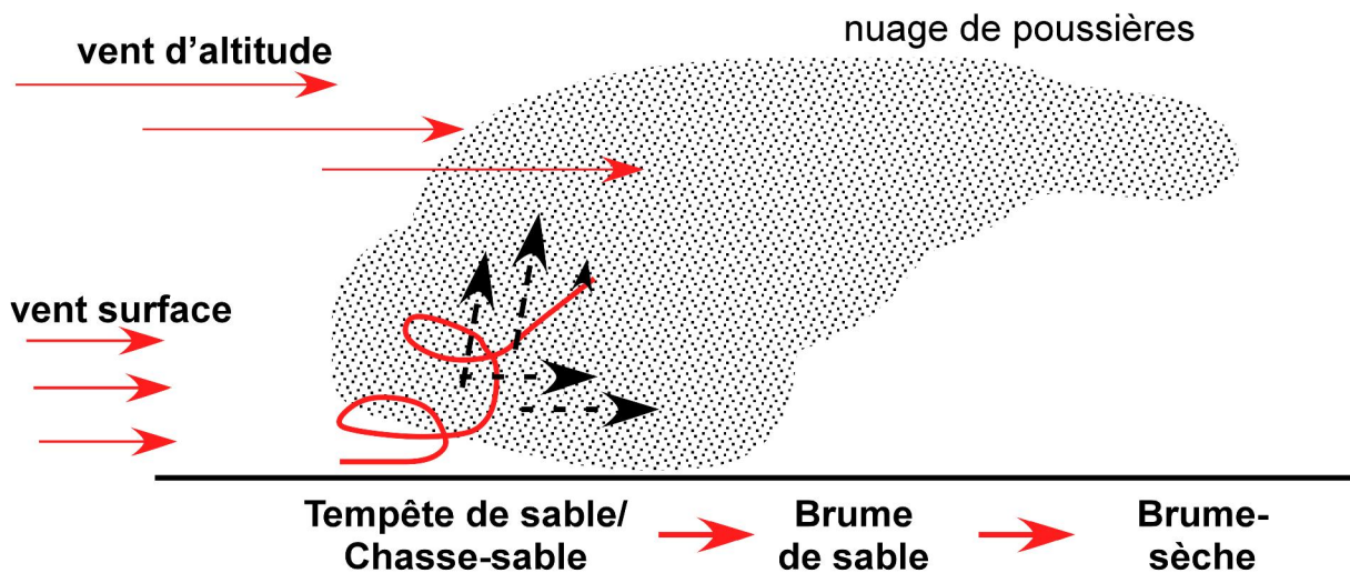
Schéma : Types de tempêtes météorologiques liés à la baisse de la visibilité horizontale
