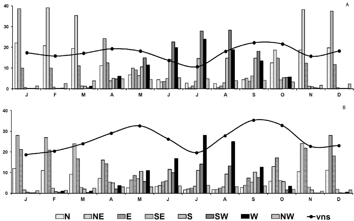
Figure 29 : Proportion mensuelle des principales directions de vent observées à 6h, 12h et 18h et des observations sans vent significatif (courbe) à Maïné-Soroa (a) et Nguigmi (b) de 1950 à 1992.
