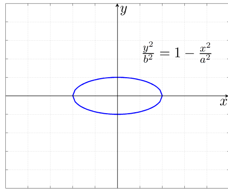
(b) Ellipse
