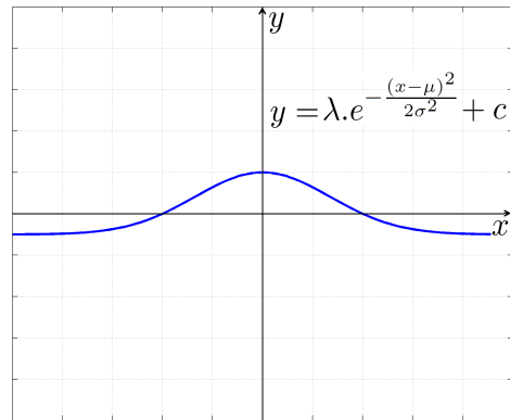
(d) Gaussian
