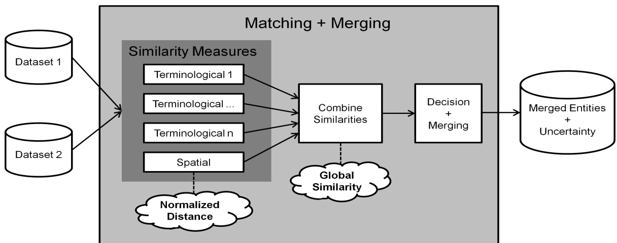
FIGURE A.5: Flux de processus de l’alignement et de fusion.
