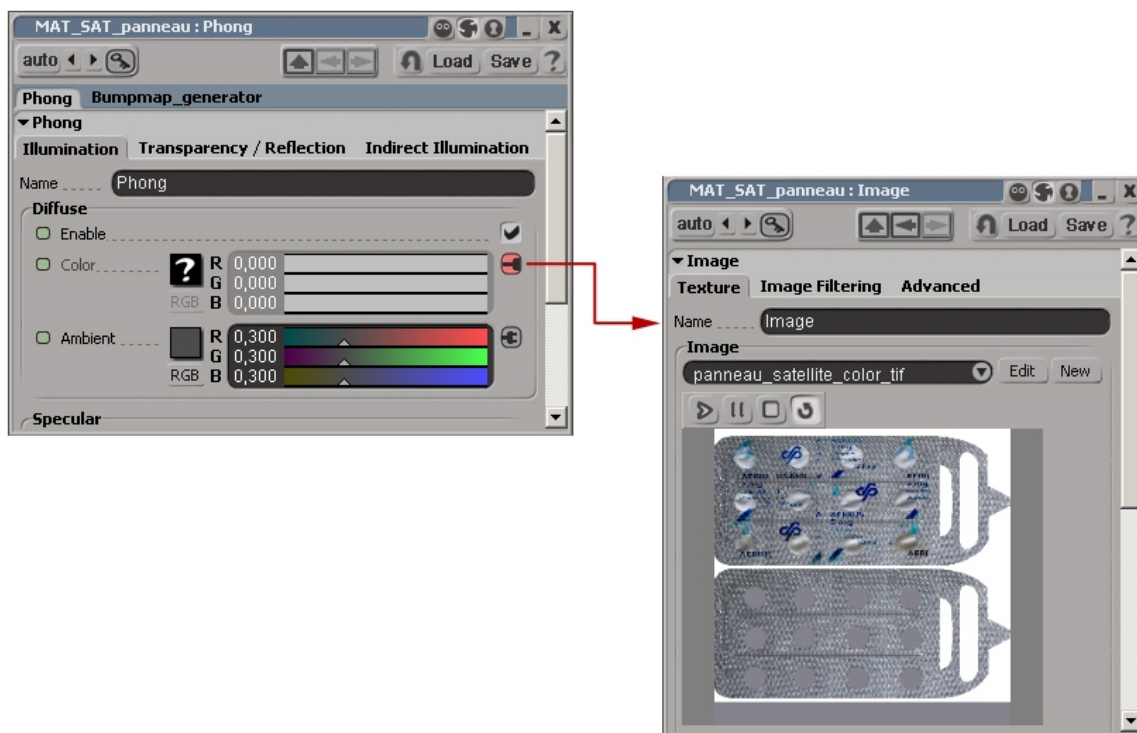
Shader dont la couleur dépend d'une image (logiciel Softimage XSI )
