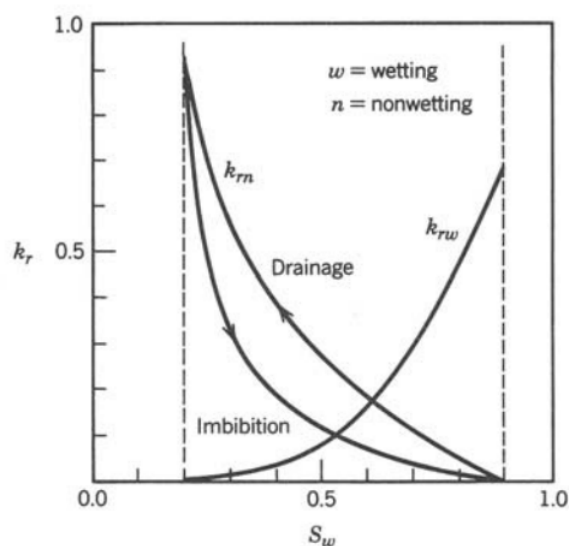
FIGURE 1.5 : Courbes de perméabilités relatives typiques (d'après [? ]).
