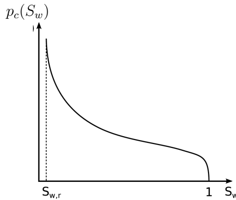
FIGURE 1.6 : Évolution de la pression capillaire en fonction de la saturation d'eau avec S_{w,r} la saturation résiduelle de l'eau selon la définition de Van Genuchten dans(??)
