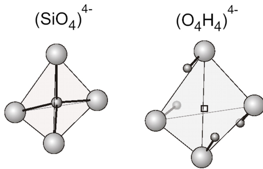
Figure I.3 – Structure d'un tétraèdre \text{SiO}_4 , ainsi que d'un tétraèdre où un site vacant de silicium a permis l'incorporation de 4 H.
