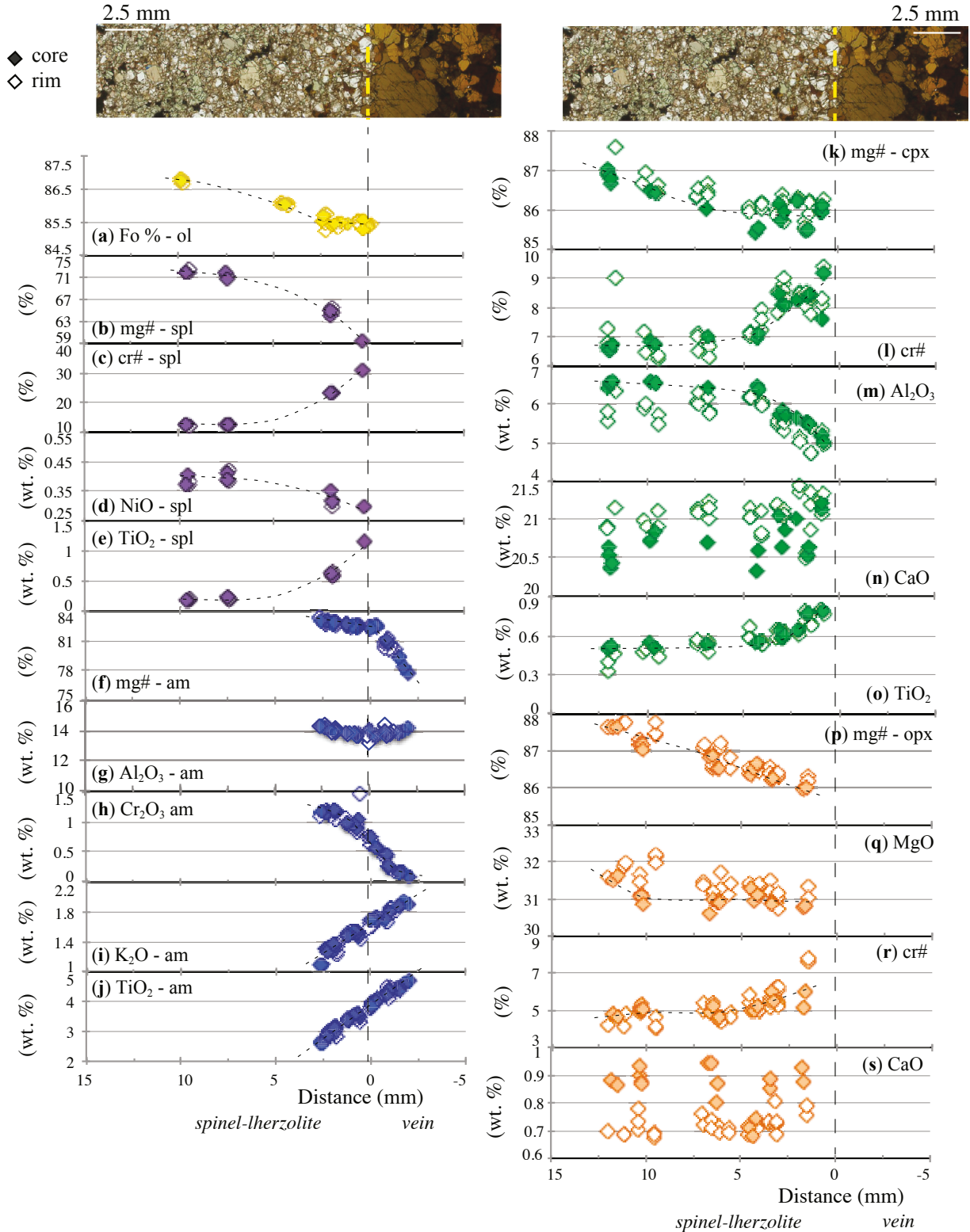
(3) Variations notables de concentration en éléments majeurs de chaque phase minérale en fonction de la distance au contact. ol : olivine ; spl : spinelle ; cpx : clinopyroxène ; opx : orthopyroxène ; am : amphibole. Fo% = 100* (Mg / (Mg + Mn+ Fe tot )) ; mg# = 100* (Mg / (Mg + Fe tot )) ; cr# = 100* (Cr / (Cr+Al tot )).
