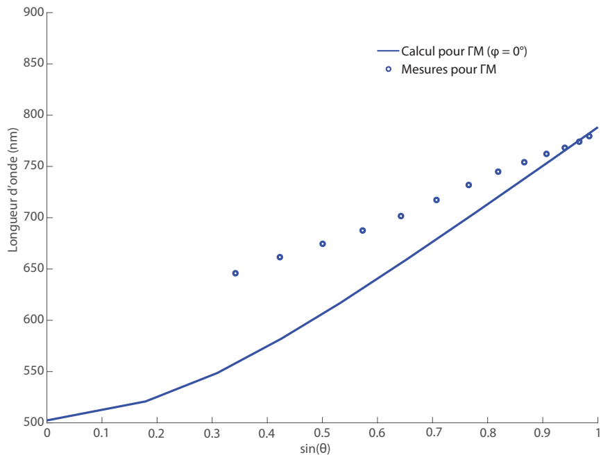
FIGURE 3.4 – Tracé des longueurs d'onde de couplage du mode \Gamma M ( \varphi = 0^\circ ) en fonction du sinus de l'angle d'incidence \theta . Les points expérimentaux mesurés avec l'expérience de réflectivité spéculaire pour un faisceau incident polarisé p ont été rajoutés en bleu pour une orientation de l'échantillon selon \Gamma M .
