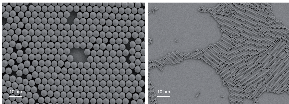
FIGURE 2.9 – Images de microscopie électronique de monocouches métallisées avec de l'or dans le cas de billes de polystyrène d'un diamètre de 5 µm (à gauche) et d'un diamètre de 1.1 µm (à droite).
