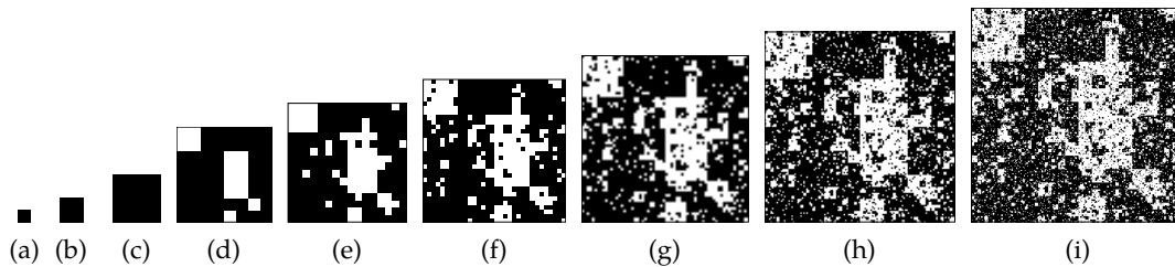
FIGURE 4.7 – Réalisation d'un arbre de Markov à deux classes et à 9 résolutions. De gauche à droite, les résolutions occupent 1, 2^2, 4^2, \dots, 256^2 pixels (échelle non respectée).
