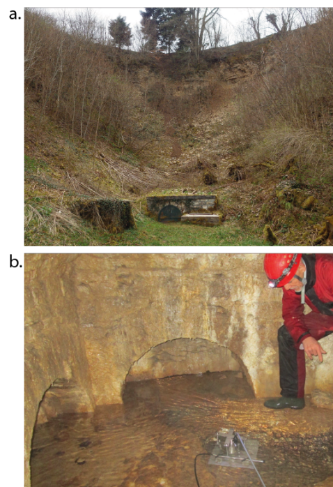
FIGURE II.14 – Captage de la source du Dahon (a) et fond du captage avec les arrivées d'eau (b)
