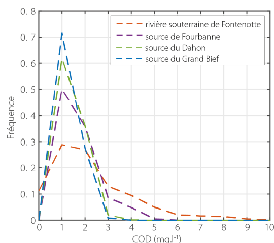
FIGURE III.11 – Fréquences de distribution de suivi semi-quantitatif du COD* pour des valeurs entre 0 et 10 \text{ mg} \cdot \text{L}^{-1} et des classes de 1 \text{ mg} \cdot \text{L}^{-1}
