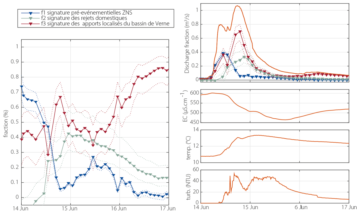
FIGURE IV.14 – Évolution de la contribution de chacun des pôles au cours de la crue de juin 2015 dans la rivière souterraine de Fontenotte avec les incertitudes associées (en pointillées) et en relation avec les paramètres physico-chimiques mesurés.
