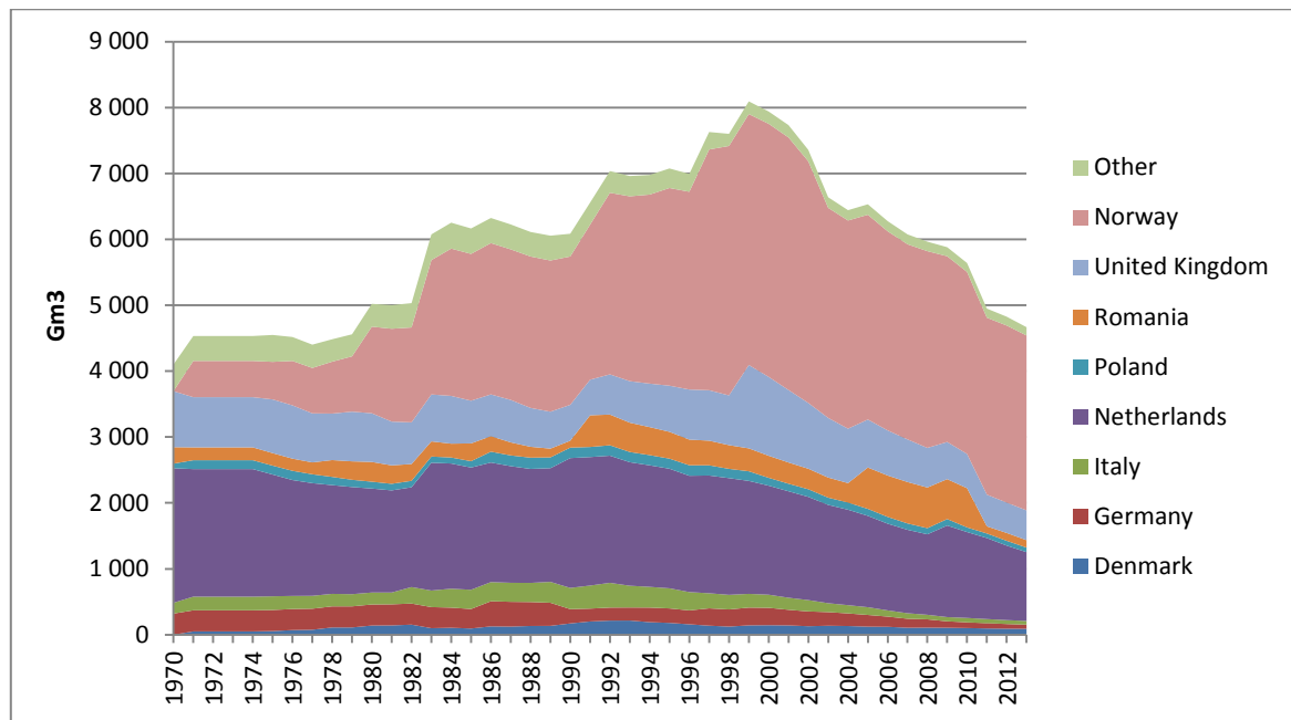
Figure 1.23 : L'évolution des réserves prouvées en Europe
