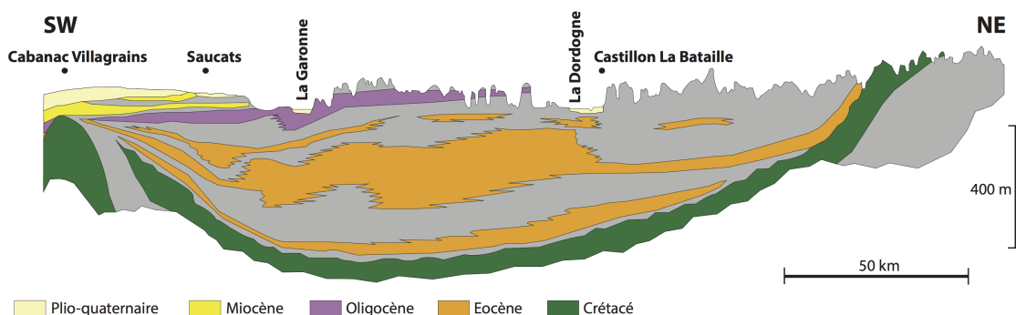
FIGURE 1: Coupe orientée NE-SW du bassin nord aquitain faisant apparaître les cinq principaux aquifères du bassin hydrogéologique. Modifié d’après Malcuit [2012].
