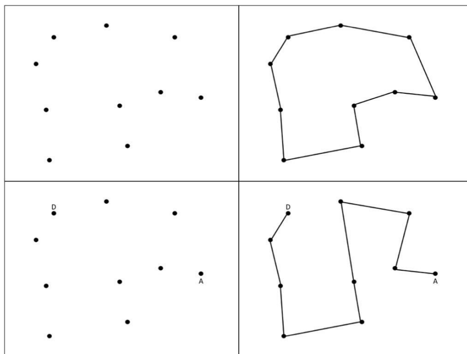
Figure 2. Exemple du problème du voyageur de commerce dans la version visuelle. En haut la version fermée est présentée, à gauche avant résolution et à droite un exemple de résolution. En bas une version ouverte est présentée, avec un « D » pour le départ et un « A » pour le point d'arrivée, à gauche le problème non résolu et à droite un exemple de résolution.
