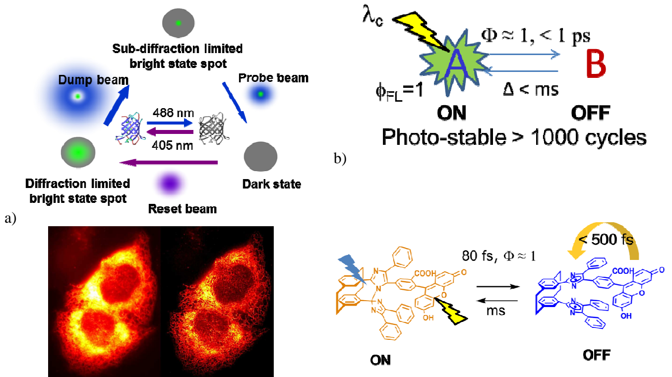
Figure 36 : b) Exemple de microscopie RESOLFT utilisant des protéines photo-réversibles [MS 14 Citation 84] et images RESOLFT utilisant la rsEGFP2 51 b) Propriétés photo-physiques nécessaires pour réaliser de la microscopie fs RESOLFT et exemple de molécules [MS 55 Citation 19].
