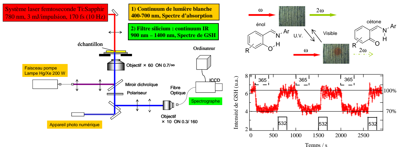
Figure 6 :Schéma du montage d'étude de la GSH en fonction de la longueur d'onde, de la photo-modulation de la GSH pour les anils et exemple de mesure de la GSH à 953 nm pendant différents cycles d'irradiation UV (énol→cétone) – visible (cétone→énol) pour un film polycristallin orienté de 4P.
