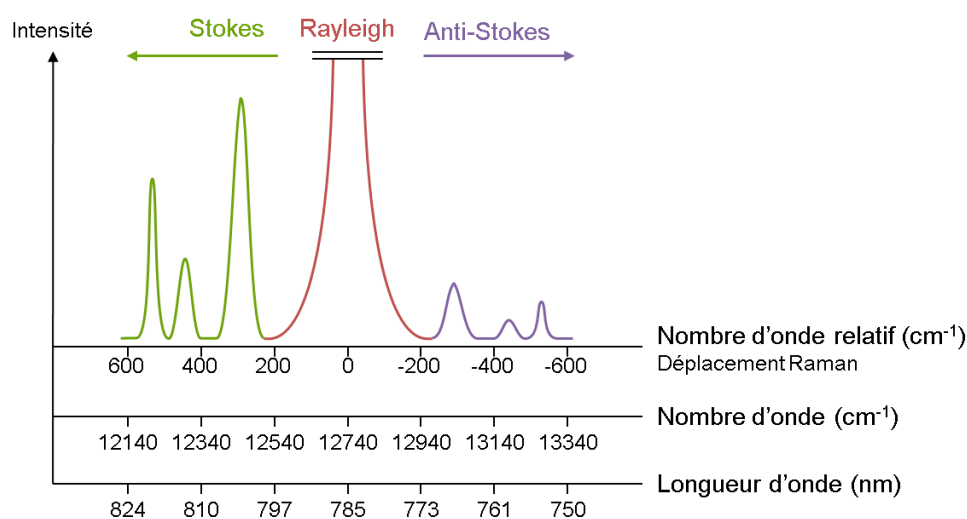
Figure 2.2 Représentation d'un spectre de diffusion. La source est un faisceau monochromatique de longueur d'onde 785 nm.
