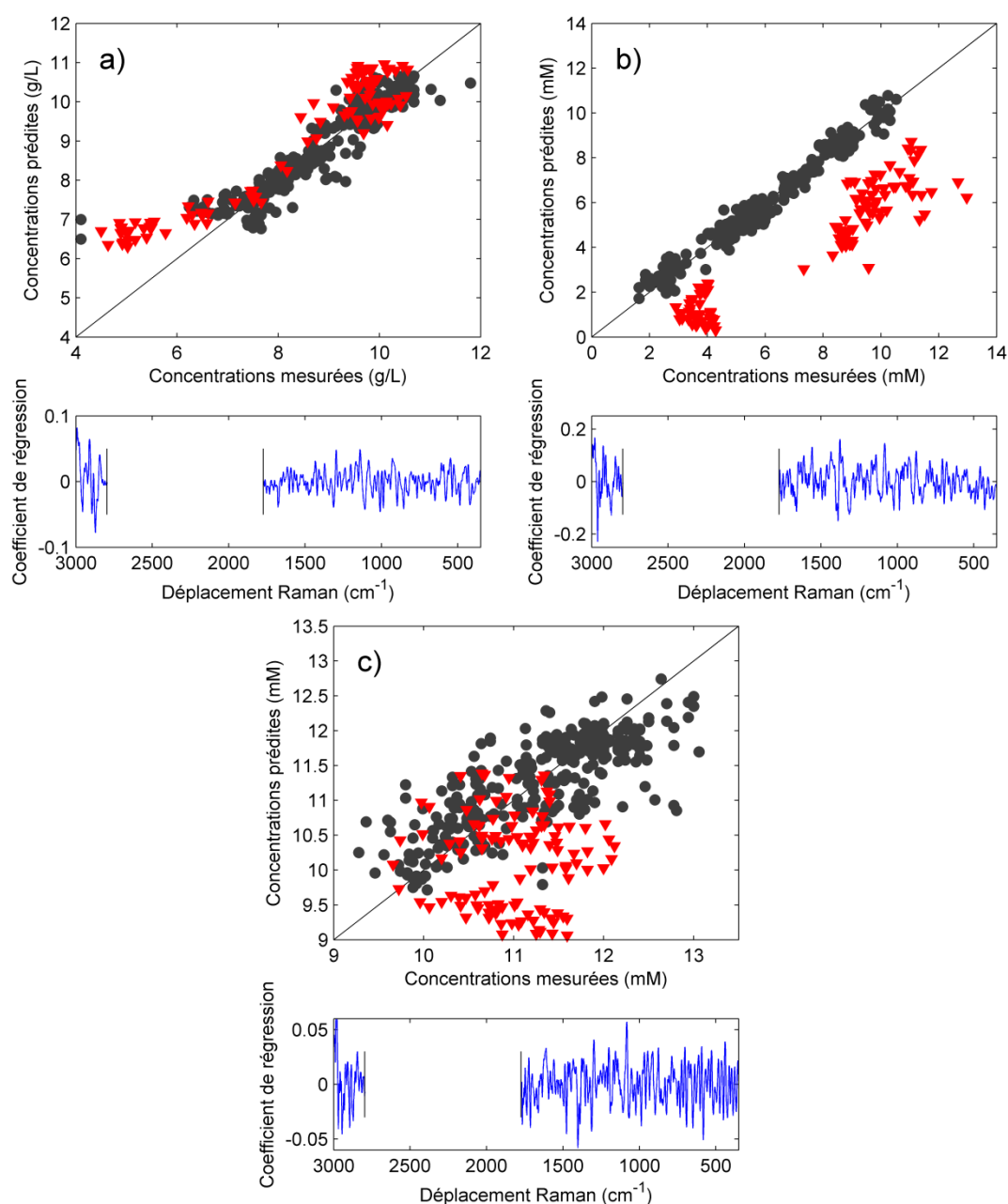
Figure 4.22 Représentations graphiques des modèles calculés à partir de jeux de données cumulant les échantillons de plusieurs lots d'amplifications cellulaires et de cultures virales mettant en jeu les cellules Sf9 pour les concentrations a) en glucose, b) en glutamine et c) en glutamate. Les points noirs représentent les échantillons de calibration, les triangles rouges les échantillons du jeu test.
