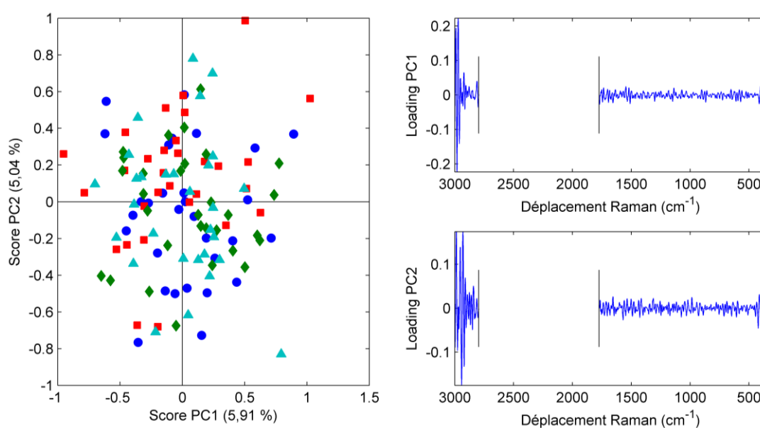
Figure 3.22 Représentation du modèle ACP réalisé sur les 120 spectres acquis pour l'étude du montage de la tête de sonde. Le prétraitement des spectres est une dérivée première suivie d'une normalisation SNV, puis sélection des régions spectrales 3000\text{--}2800\text{ cm}^{-1} et 1775\text{--}350\text{ cm}^{-1} . Sur le graphique des scores (à gauche), les points bleus représentent l'opérateur #1, les carrés rouges l'opérateur #2, les losanges verts l'opérateur #3 et les triangles cyans l'opérateur #4.
