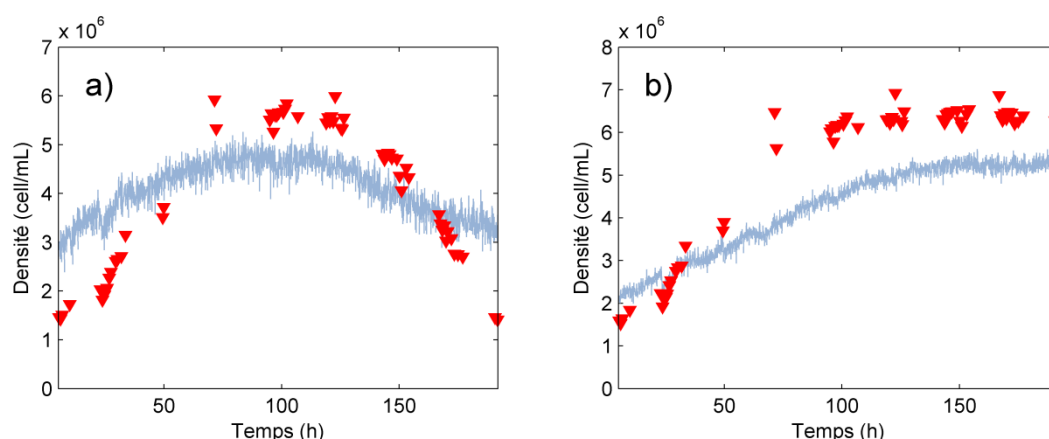
Figure 4.27 Représentations des prédictions réalisées sur les spectres de la culture de cellules Sf9 #4 acquis en continu (en cyan) pour a) la densité VCD et b) la densité TCD durant la phase de culture virale. Les densités obtenues à partir des mesures de référence sur les prélèvements sont représentées par les triangles rouges.
