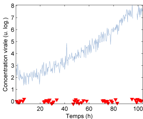
Figure 5.5 Prédictions de la concentration en virus (en bleu) réalisées sur les spectres acquis en continu de la culture de cellules #1-1. Les mesures références (triangles rouges) sont créées artificiellement autour de 0,00 u. log., en prenant en compte l'erreur de la méthode de référence de manière aléatoire.
