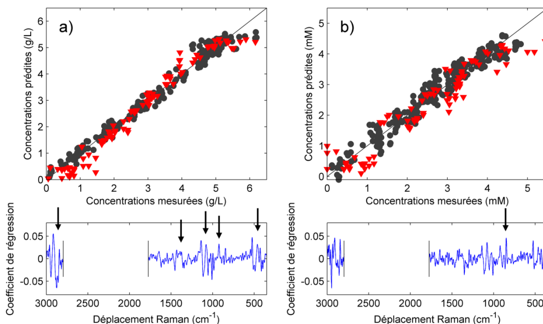
Figure 4.9 Représentations graphiques des modèles calculés à partir de jeux de données cumulants les échantillons de plusieurs cultures de cellules HeLa pour les concentrations a) en glucose et b) en glutamine. Les points noirs représentent les échantillons de calibration, les triangles rouges les échantillons du jeu test.
