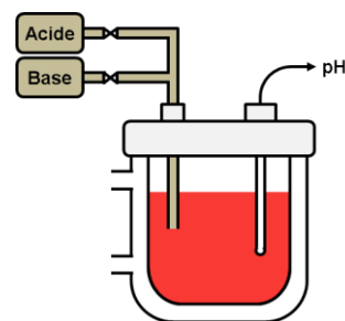
Figure 1.15 Schéma du dispositif de contrôle du pH.
