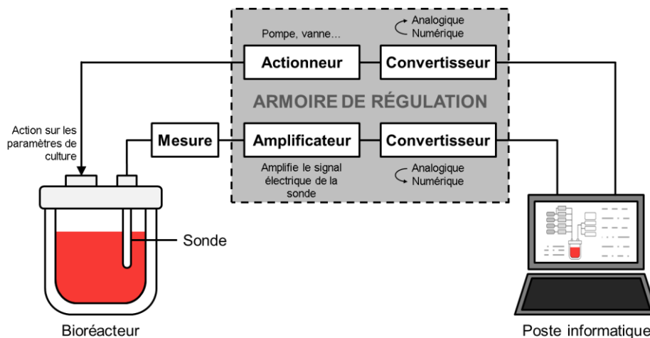
Figure 1.13 Représentation du système de régulation des paramètres : Set Point Control .
