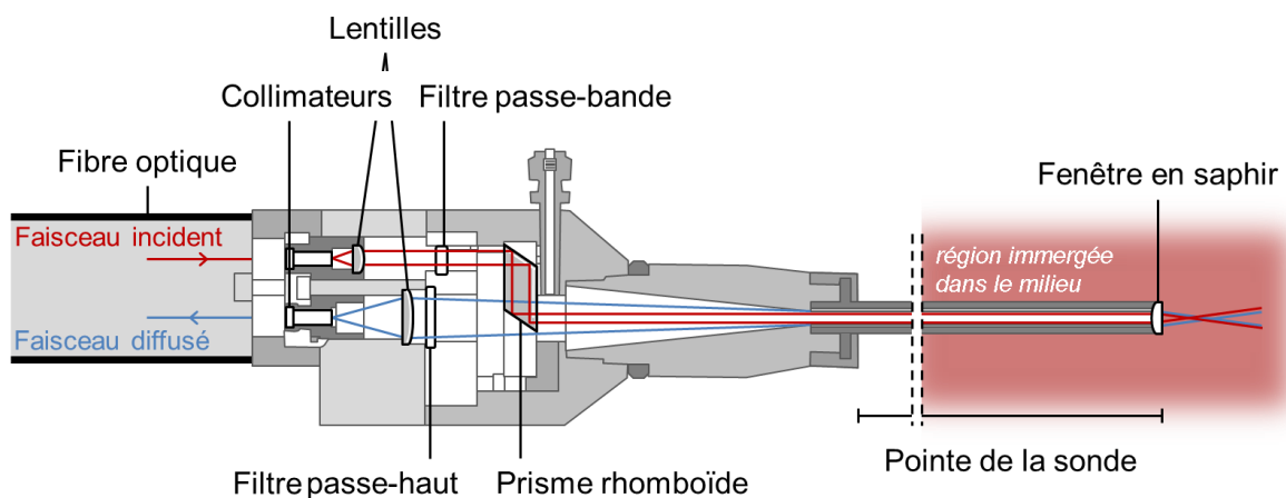
Figure 2.4 Représentation d'un exemple de montage de la tête de sonde à immersion Raman [62].
