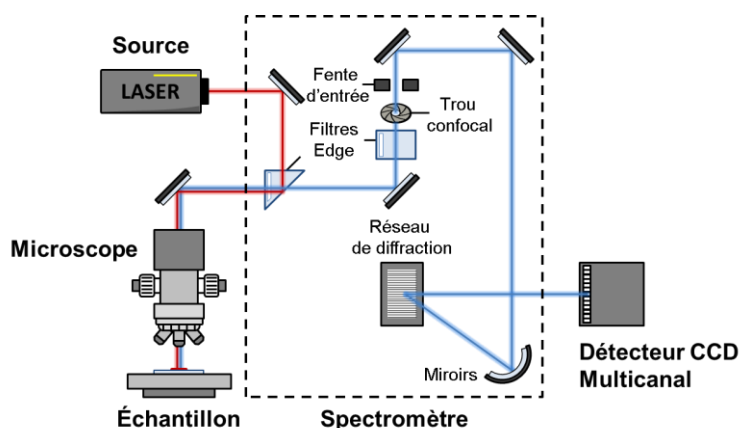
Figure 2.3 Représentation schématique d'un microspectromètre Raman.
