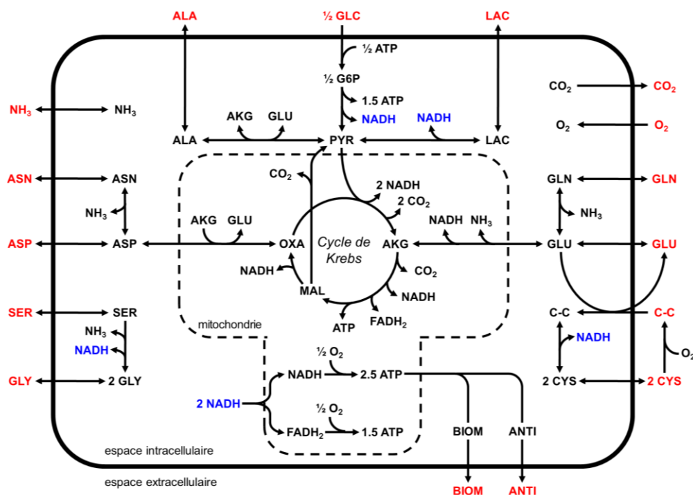
Figure 1.4 Schéma du métabolisme des cellules mammifères. Les métabolites extracellulaires sont représentés en rouge tandis que les métabolites intracellulaires sont représentés en noir, tout comme les molécules NADH mitochondriales. Les molécules NADH cytosoliques (présents dans le liquide cytoplasmique des cellules) sont représentées en bleu [4]. AKG : \alpha -cétoglutarate, ALA : Alanine, ANTI : Antibody concentration , ASN : Asparagine, ASP : Aspartate, ATP : Adénosine triphosphate, BIOM : Biomasse, CYS : Cystéine, FADH 2 : Flavine adénine dinucléotide, G6P : Glucose-6-phosphate, GLC : Glucose, GLN : Glutamine, GLU : Glutamate, GLY : Glycine, MAL : Malate, NADH : Nicotinamide adénine dinucléotide, NH 3 : Ammoniac, OXA : Oxaloacétate, PYR : Pyruvate, SER : Sérine.
