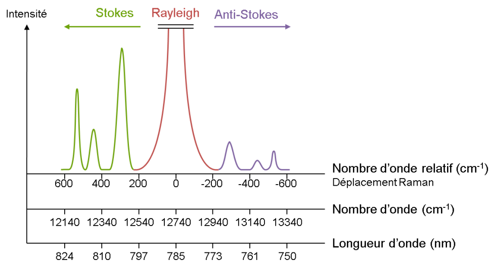
Figure 2.2 Représentation d'un spectre de diffusion. La source est un faisceau monochromatique de longueur d'onde 785 nm.
