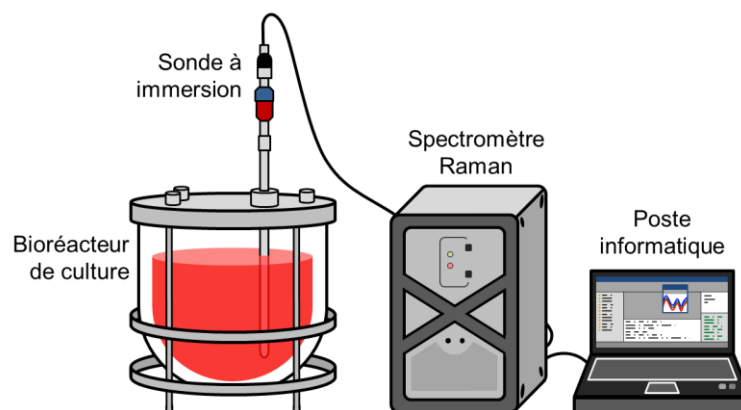
Figure 3.1 Représentation du montage pour le suivi Raman d'une culture cellulaire. La sonde à immersion reliée au spectromètre Raman est fixée à la platine du bioréacteur et plongée au sein du milieu de culture. Le poste informatique permet de régler les paramètres spécifiques à l'acquisition des spectres Raman.
