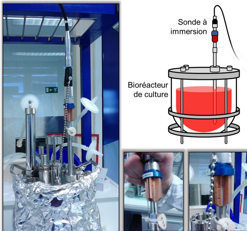
Figure 3.20 Représentation du montage de la sonde à immersion sur le bioréacteur de culture. Les vues rapprochées permettent de mettre en avant le repère gris pour l'alignement des fibres optiques de la tête et du corps de la sonde Raman.
