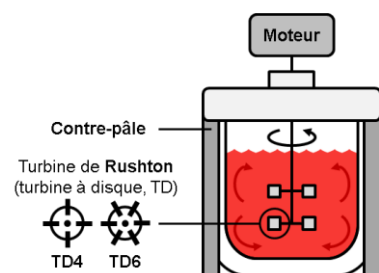
Figure 1.17 Schéma du dispositif d'agitation radiale.
