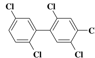
2,4,5,2',5'-Pentachlorobiphényle (CB101)
