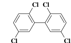
2,5,2',5'-Tetrachlorobiphényle (CB52)
