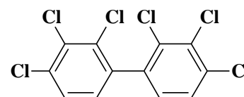
2,3,4,2',3',4'-Hexachlorobiphényle (CB128)
