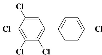
2,3,4,4',5-Pentachlorobiphényle (CB114)
