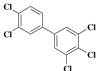
3,4,5,3',4'-Pentachlorobiphényle (CB126)
