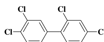
2,3',4,4'-Tetrachlorobiphényle (CB66)
