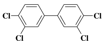
3,4,3',4'-Tetrachlorobiphényle (CB77)
