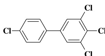
3,4,4',5-Tetrachlorobiphényle (CB81)
