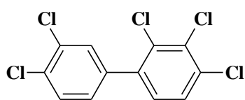
2,3,3',4,4'-Pentachlorobiphényle (CB105)
