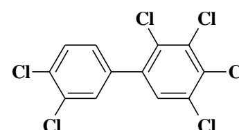
2,3,3',4,4',5-Hexachlorobiphényle (CB156)
