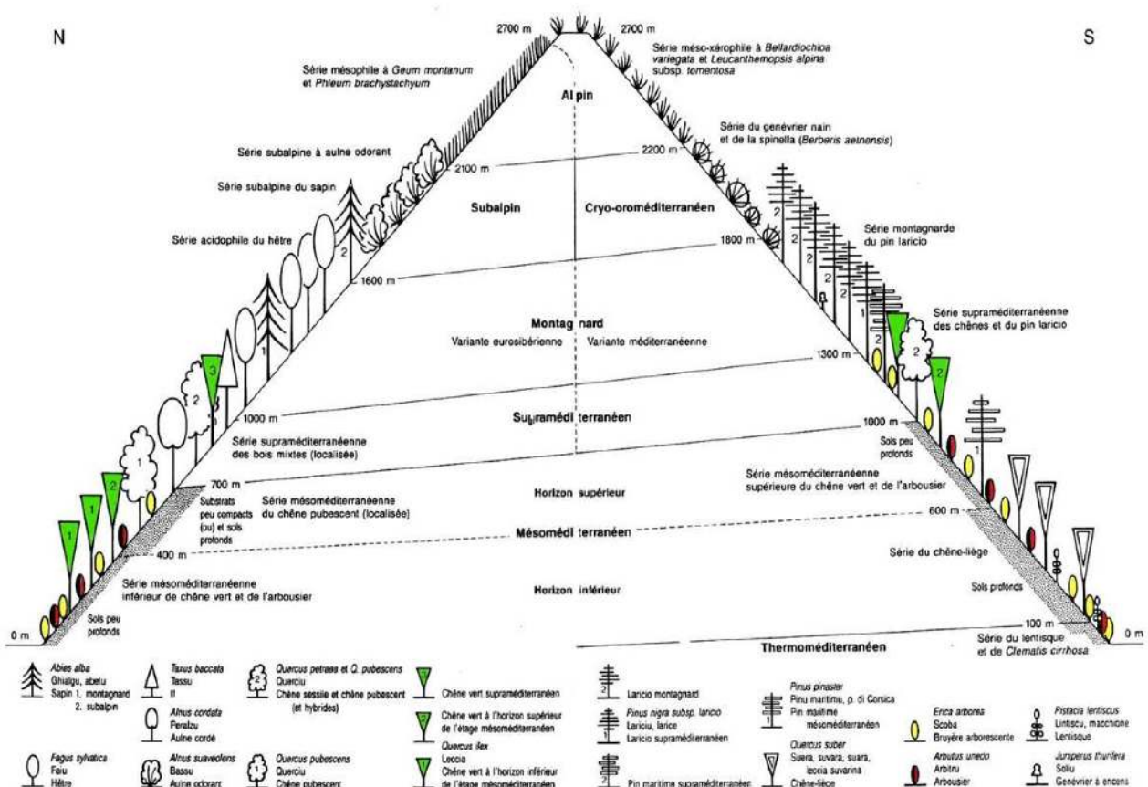
FIGURE I.18 – Étages de végétation en Corse et répartition des principales espèces végétales structurant les écosystèmes (à partir de Gamisans 1999).
