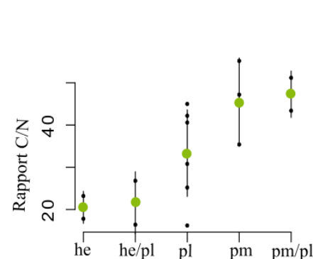
Figure 7 – Rapport carbone/azote en fonction des modalités de coexistences.
