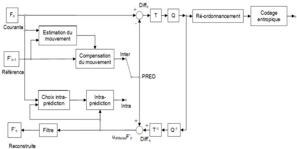
FIGURE 2.9. Encodeur H.264
