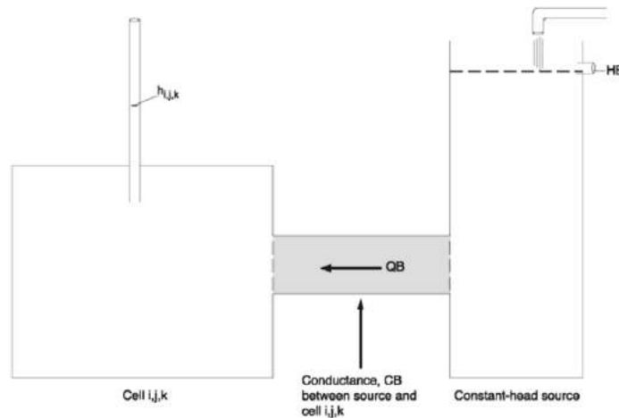
Figure 5.4 : Fonctionnement de la condition limite de type GHB d'après McDonald and Harbaugh (1988)
