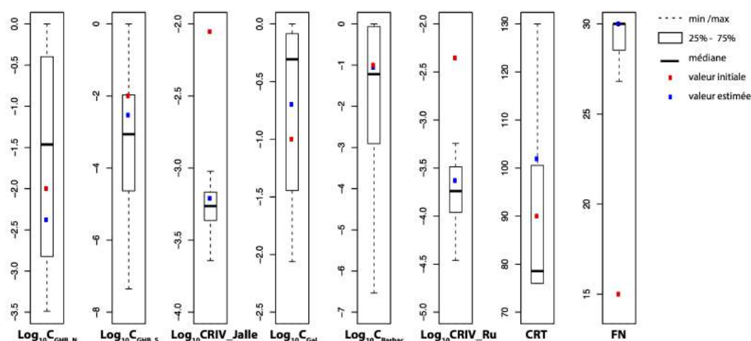
Figure 7.19 : Diagramme en boîte de la répartition obtenue de chaque paramètre par la méthode NSMC. C_{GHB_N} et C_{GHB_S} sont les conductance des conditions limites nord et sud, CRIV\_Jalle et CRIV\_Ru sont les coefficients rivière des conditions limites rivière de la Jalle et du ruisseau Ste Christine, C_{galerie} et C_{Barbacanes} sont les conductances des drains (Galerie de Gamarde et Barbacanes), CRT la capacité au champ moyenne et FN la capacité d'infiltration du sol sont les paramètres de la fonction de production de Ledoux (Ledoux et al., 1984).
