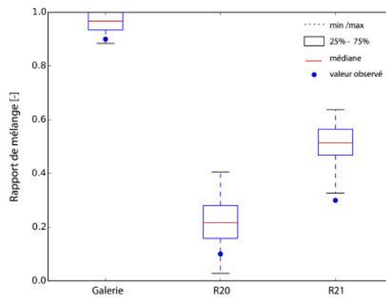
Figure 7.22 : Distribution des rapports de mélanges simulés aux ouvrages de productions obtenue par NSMC
