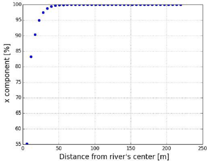
Figure 5.2 : Part horizontale de l'écoulement, tous les 5 m depuis le centre de la rivière, calculée avec l'application développée chapitre 3. Dans le cas présent, on peut considérer que les écoulements sont strictement horizontaux au delà de 50 m de la rivière
