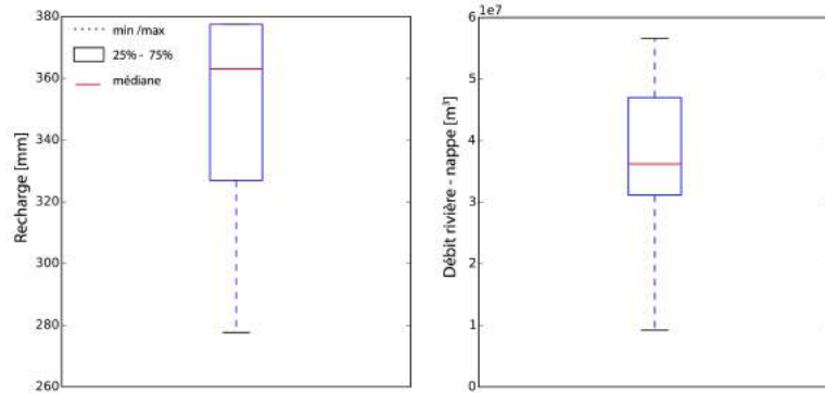
Figure 7.21 : Distribution A) de la lame d'eau de recharge et B) des volumes échangés rivière - nappe obtenus par NSMC sur la période de calibration
