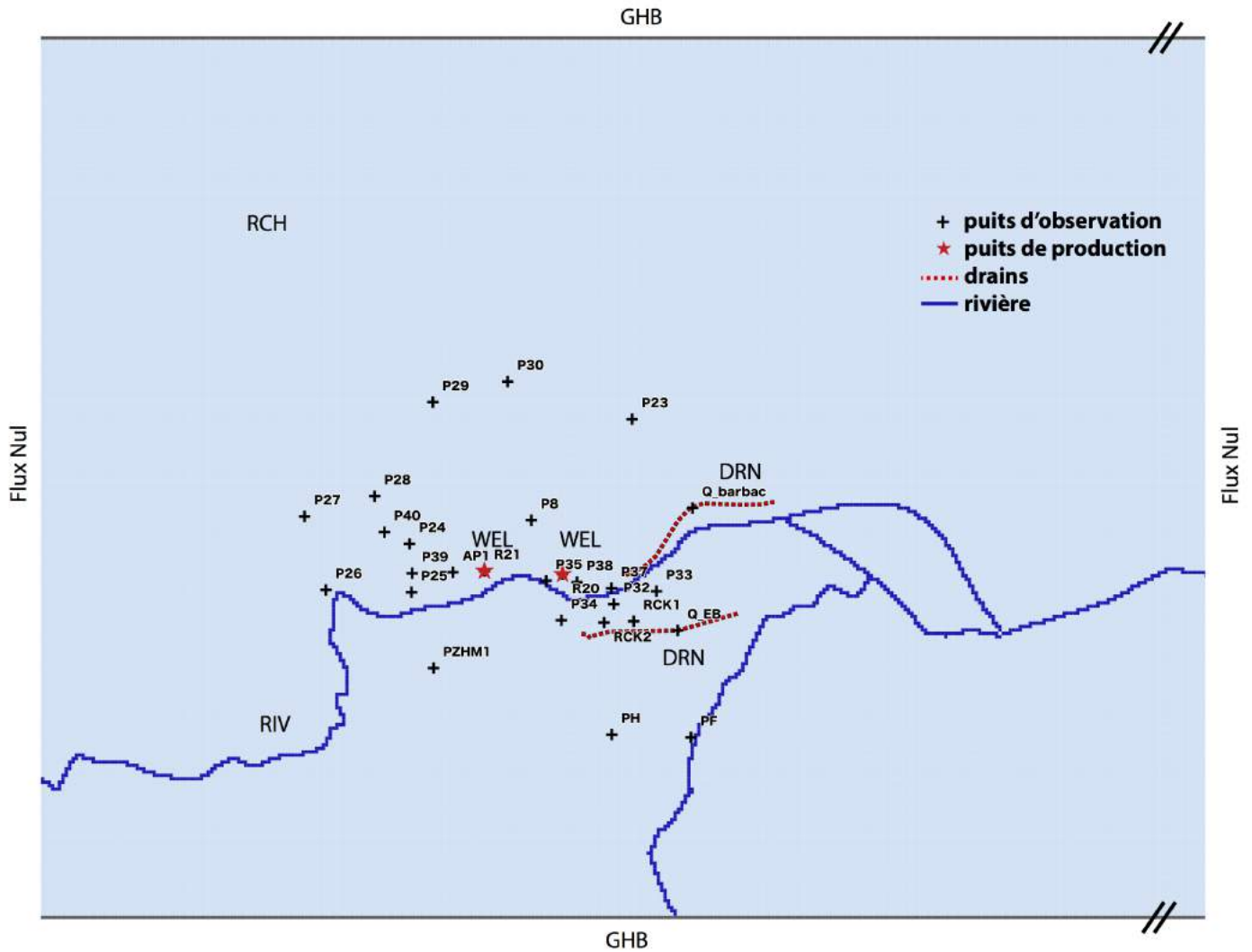
Figure 5.7 : Synthèse des conditions limites du modèle d'écoulement. A noter que par soucis de visibilité l'emprise du modèle dans sa partie est a été légèrement raccourcie.
