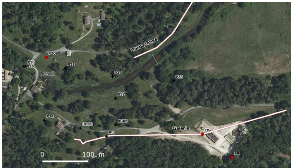
Figure 8.3 : Positionnement de la galerie de Gamarde dans le champ captant de Thil-Gamarde, avec le regard Rth, ainsi que le point de pompage EB
