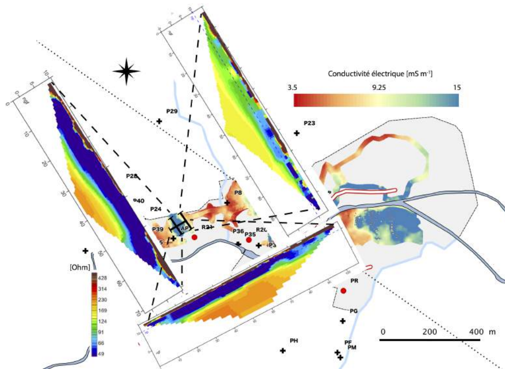
Figure 4.29 : Cartographie de conductivité électrique EM31 et profil de résistivité électrique à travers la zone conductrice dans l'alignement de l'ouvrage de production R21
