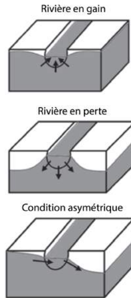
Figure 5.8 : Configuration asymétrique des échanges nappe-rivière par rapport au régime en gain et en perte de la rivière, modifié d'après Ben Simon et al. (2015)
