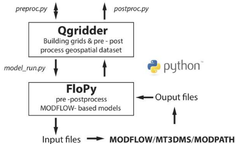
Figure 5.1 : Schéma conceptuel de la plateforme de modélisation utilisée : l'interface graphique du SIG Qgis est d'abord utilisée pour visualiser et pré-traiter les données géographiques d'entrée. Le plugin Qgis Qgriidder est alors employé pour générer le maillage. Les scripts Python preproc.py et model_run.py sont ensuite exécutés pour terminer le traitement des données d'entrée et communiquer avec le wrapper FloPy pour l'exécution d'un ou plusieurs modèles. Les résultats du modèle sont renvoyés vers Qgis pour la visualisation et le traitement, par l'intermédiaire de FloPy et du script Python postproc.py
