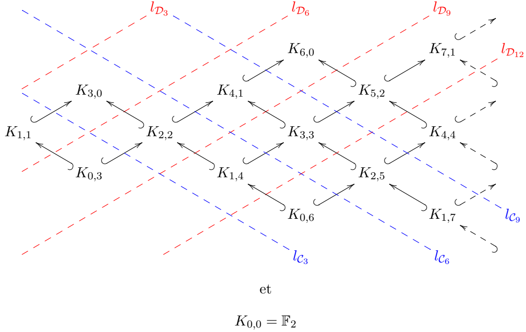
FIGURE 2.4 – Sous-foncteurs du foncteur \mathcal{K}_2^{\bar{0}} : V \mapsto K(2)^{\bar{0}}(BV^{\#}) .
