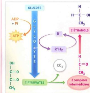
Les réactions de la fermentation alcoolique.
