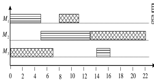
Figure III. 1 : Ordonnancement de la production
