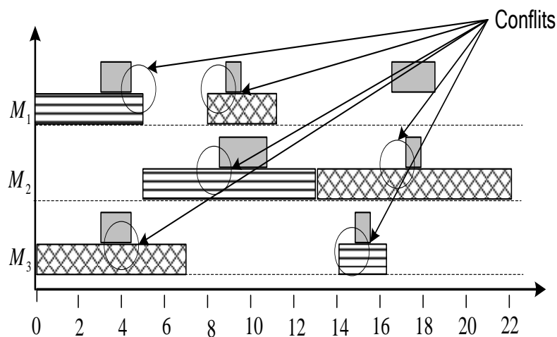
Figure III. 3 : Conflits entre tâches de maintenance et tâches de production dans un ordonnancement séparé
