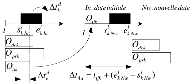
Figure III. 8 : Affection des opérations suivant la règle 4a
