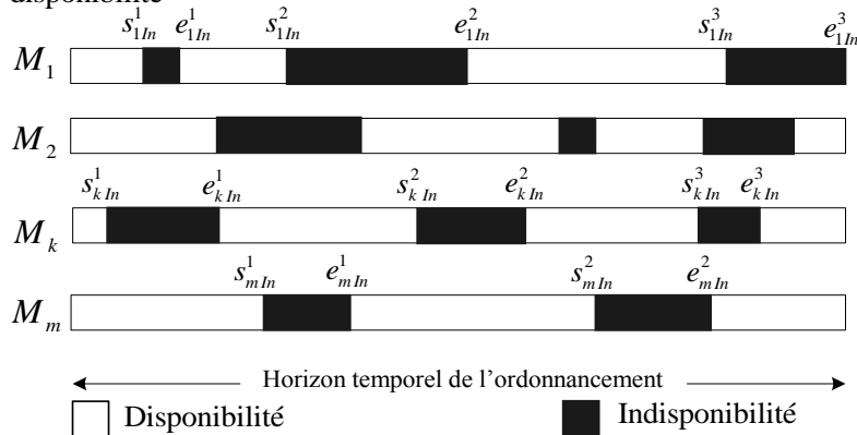
Figure III. 4 : Présentation du modèle générique du problème
