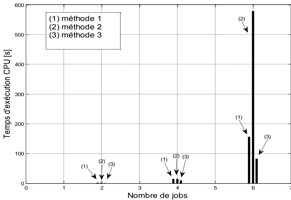
Figure II. 19 : Variation du temps d'exécution en fonction du nombre de jobs
