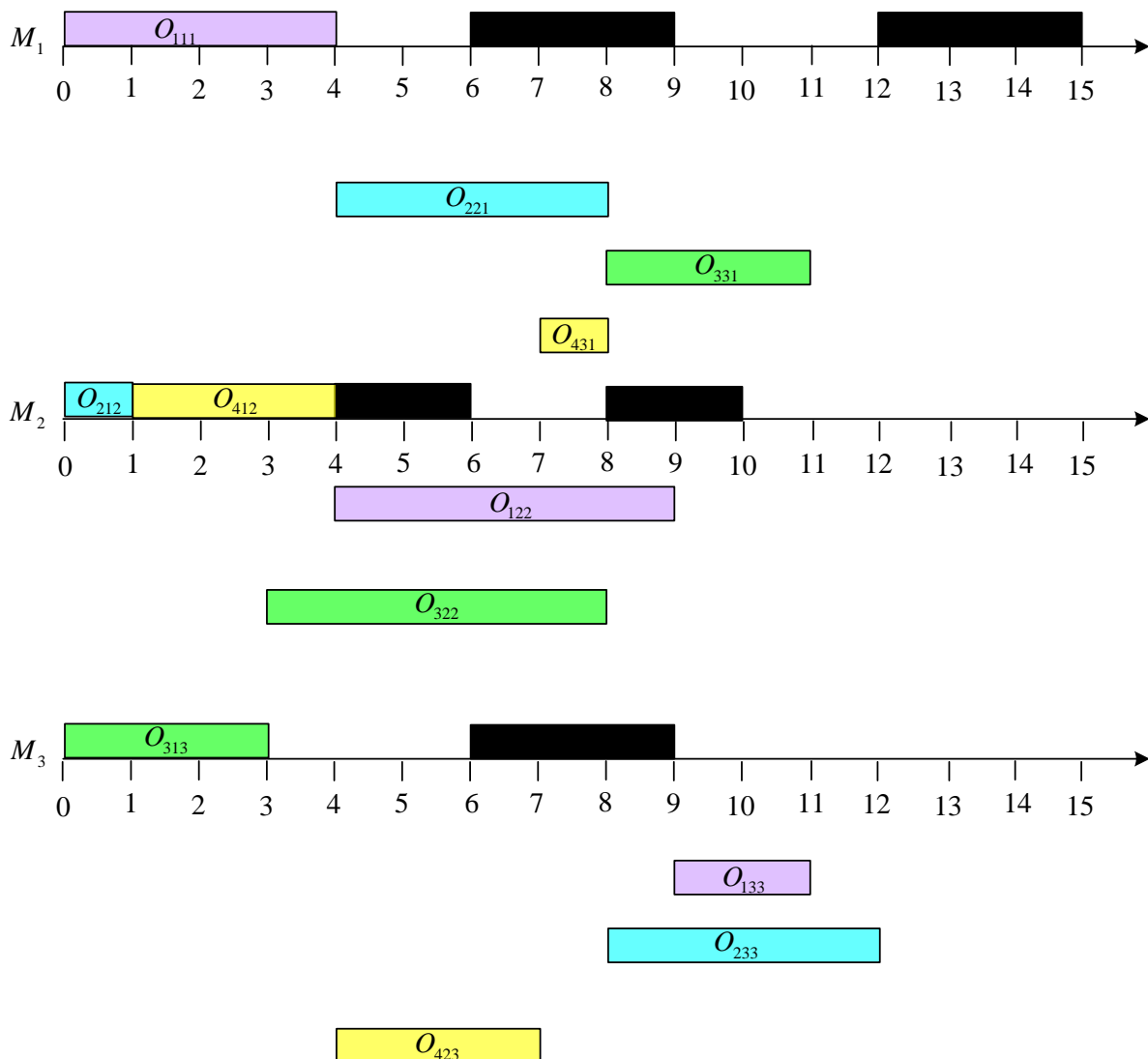
Figure III. 14 : Allocation des opérations aux machines suivant la règle 1 à l'instant t = 2
