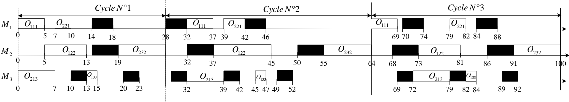
Figure III. 23 : Allocation des tâches en utilisant la nouvelle méthode de décalage
