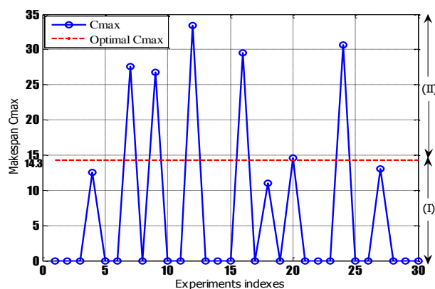
Figure II. 16 : Résultats de la simulation utilisant la méthode d'initialisation aléatoire pour l'exemple 2: 4/3/J/Cmax
