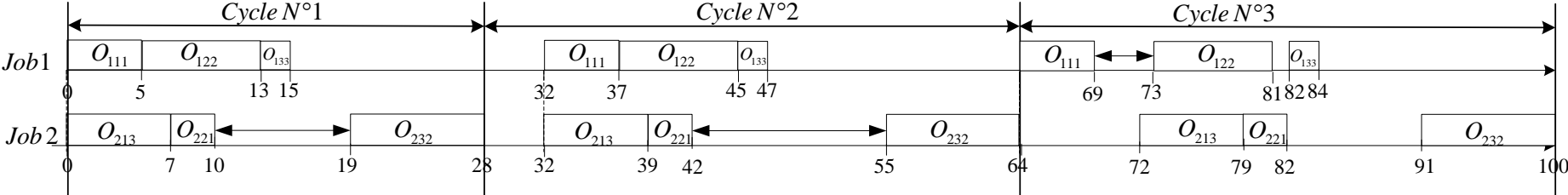
Figure III. 22 : Allocation des tâches en utilisant la nouvelle méthode de décalage
