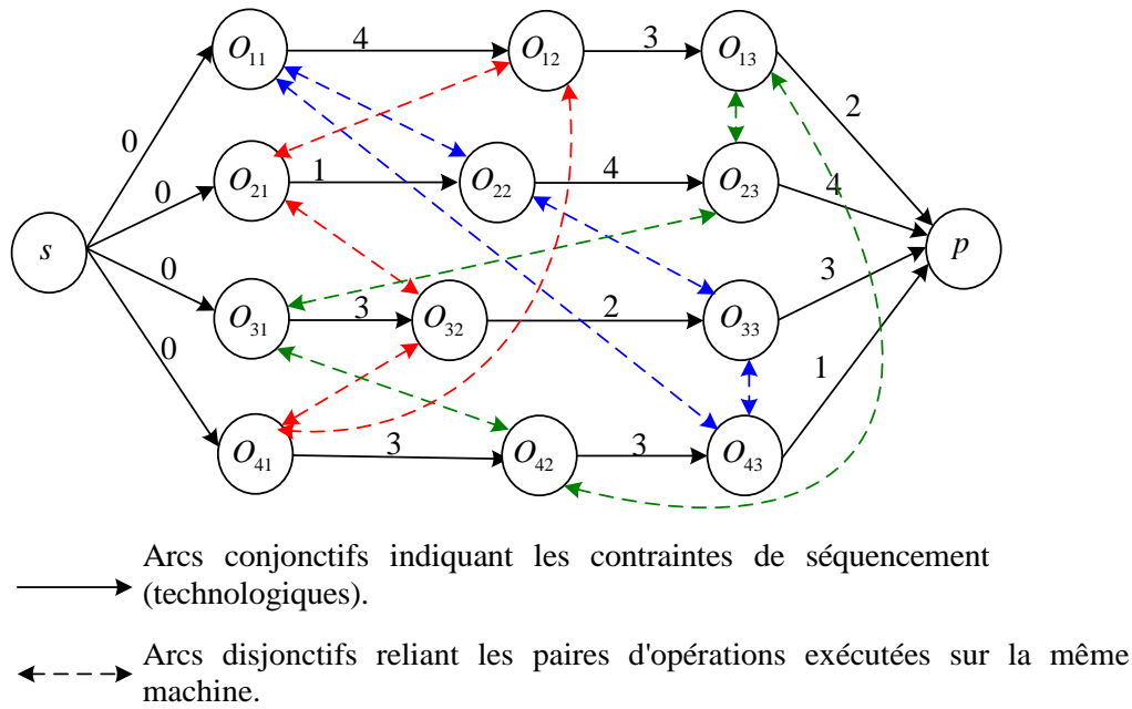
Figure I. 4 : Graphe disjonctif d'un job shop de 4 tâches et de 3 machines (Tableau I. 3)
