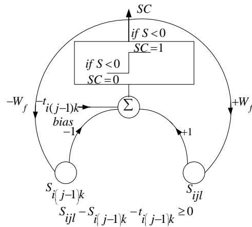
Figure II. 7 : Réseau de Hopfield illustrant les contraintes de séquençement unité-CS
