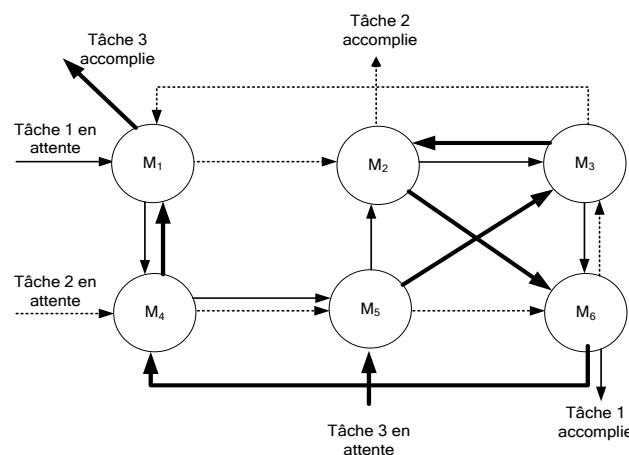
Figure I. 3 : Exemple d'un atelier de type job shop de 3 tâches et de 6 machines
