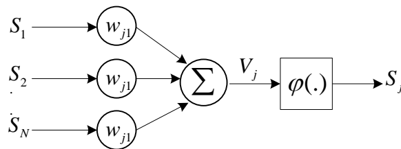
Figure II. 1 : Structure d'un neurone artificiel.
