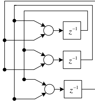
Figure II. 3 : Architecture générale d'un réseau de neurone Hopfield constitué de 3 neurones
