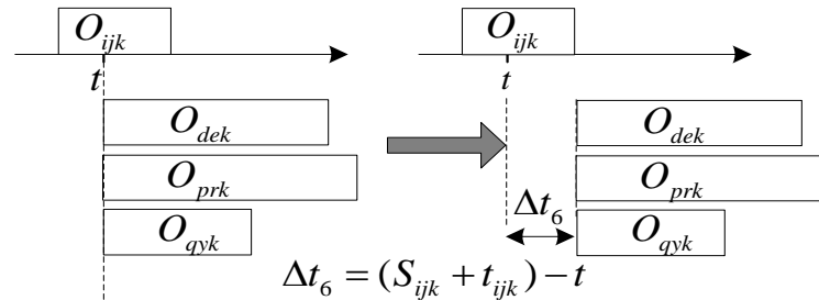
Figure III. 11 : Décalage de la liste d'attente suivant la règle 6
