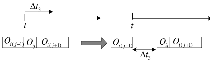
Figure III. 7 : Décalage des opérations suivant la règle 3
