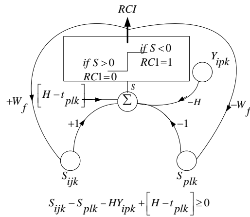
Figure II. 8 : Réseau de Hopfield illustrant les contraintes de ressources CRI
