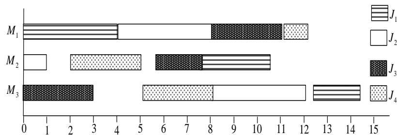
Figure I. 5 : Diagramme de Gantt visualisant un job shop de 4 tâches et de 3 machines
