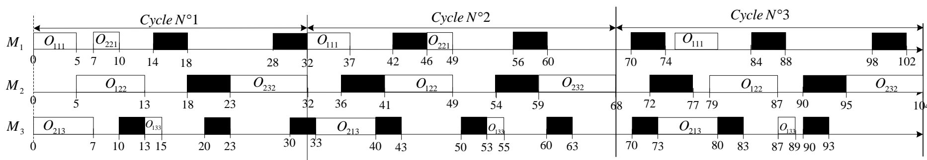
Figure III. 21 : Allocation des machines avec contraintes de tâches de maintenance (fixe)
