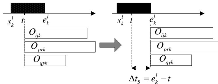
Figure III. 10 : Affection des opérations suivant la règle 5
