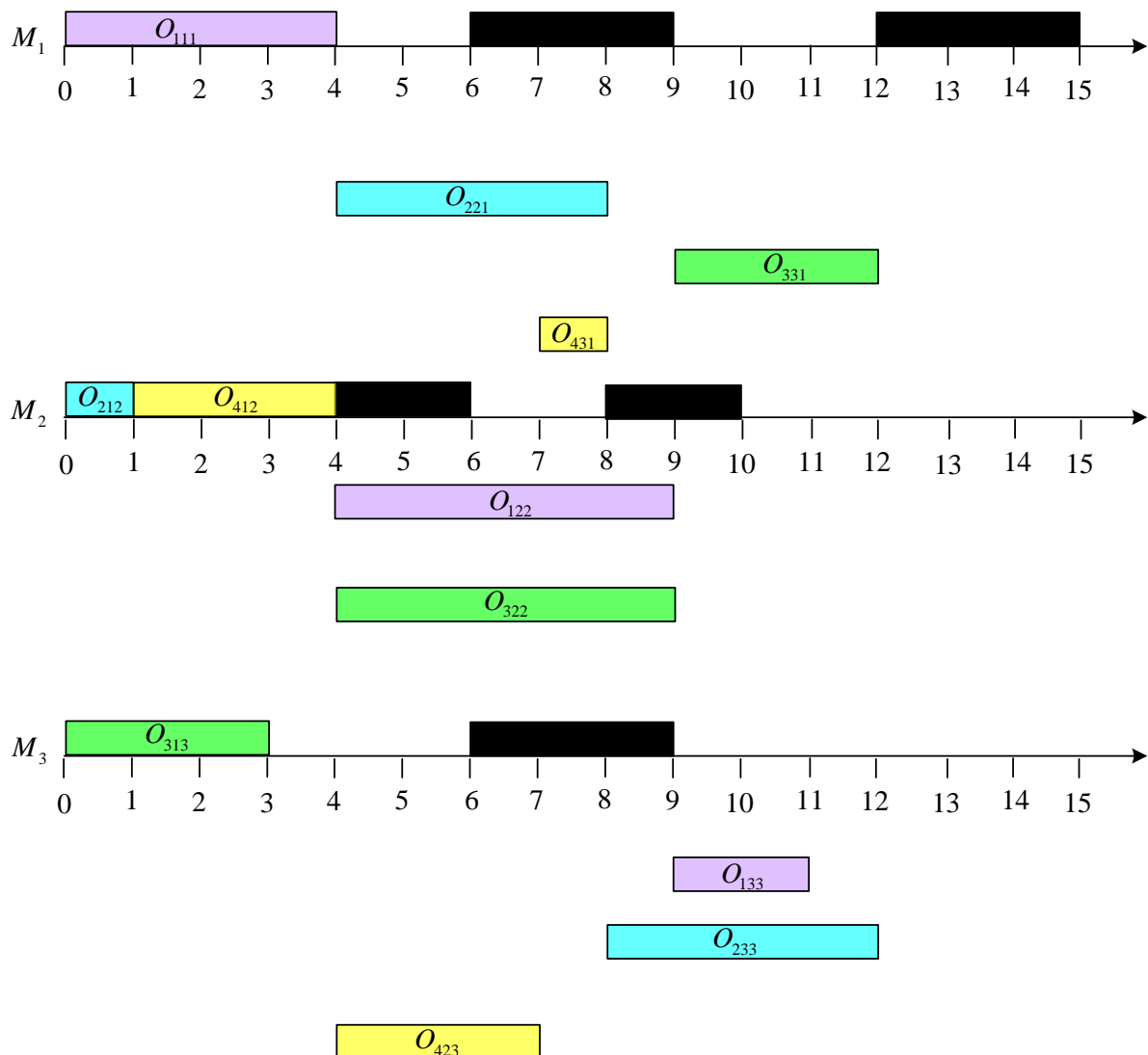
Figure III. 15 : Allocation des opérations aux machines suivant la règle 1 à l'instant t = 3
