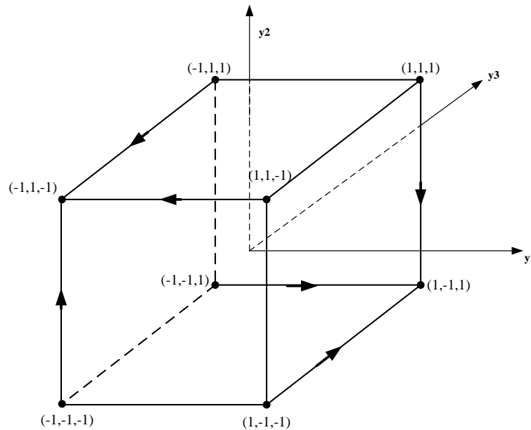
Figure II. 5 : Architecture graphique du réseau de neurone de Hopfield de 3 neurones
