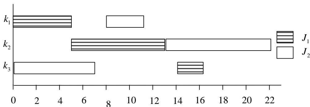
Figure II. 17 : Diagramme de Gantt correspondant à la solution du test de l'exemple 1 par la troisième méthode d'initialisation
