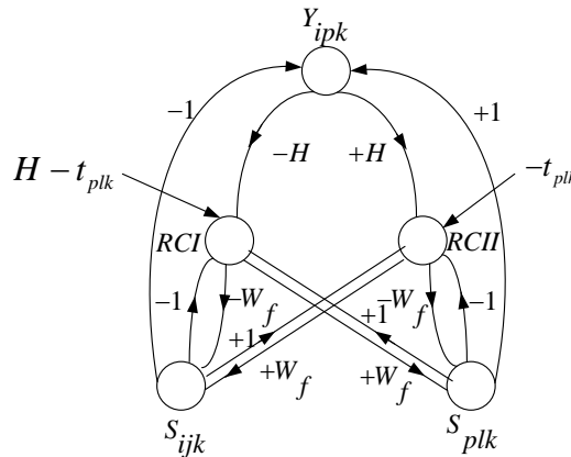
Figure II. 10 : Architecture générale des contraintes de ressources RCI et RCII
