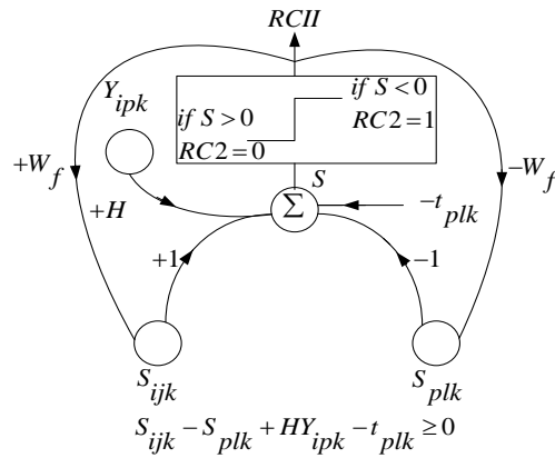
Figure II. 9 : Réseau de Hopfield illustrant les contraintes de ressources CRII
