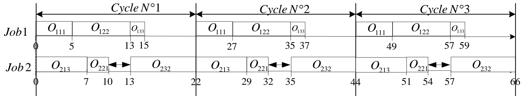
Figure III. 19 : Allocation des tâches sans contraintes de maintenance
