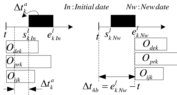
Figure III. 9 : Affection des opérations suivant la règle 4b
