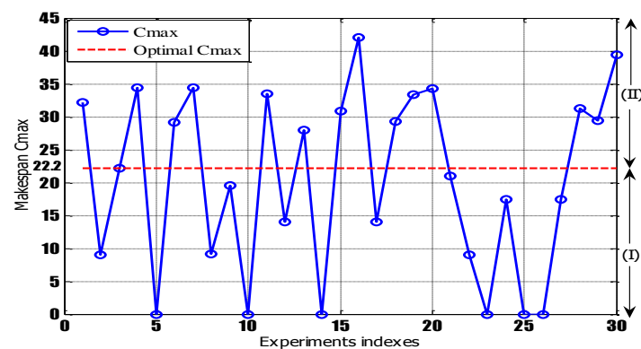
Figure II. 13 : Résultats de la simulation utilisant la méthode d'initialisation aléatoire pour l'exemple 1: 2/3/J/ C_{max}
