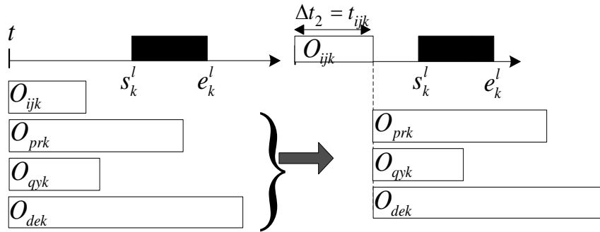
Figure III. 6 : Affection des opérations suivant la règle 2
