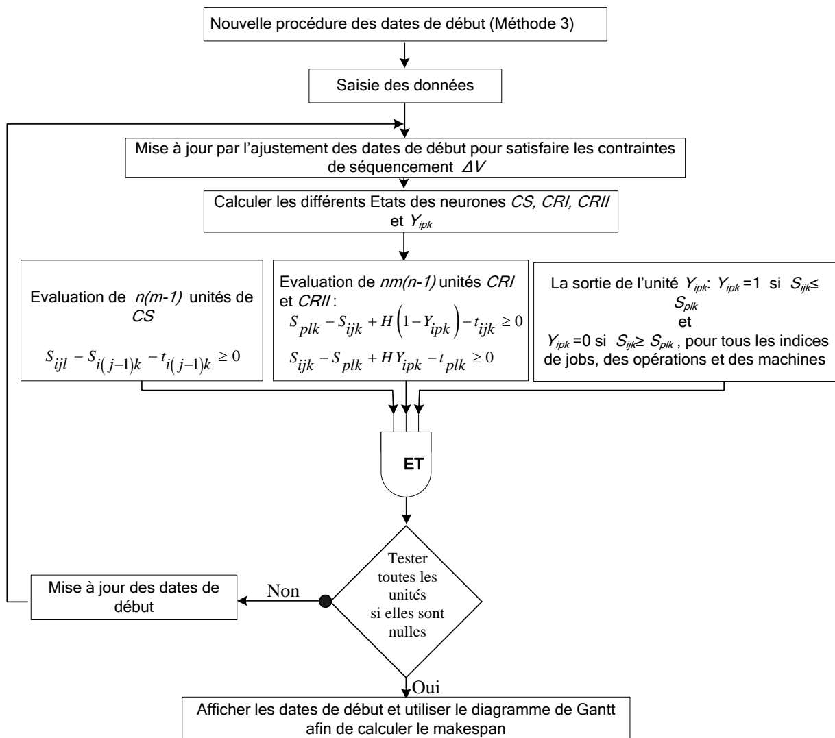
Figure II. 12 : Organigramme de l'amélioration apportée (Méthode 3)
