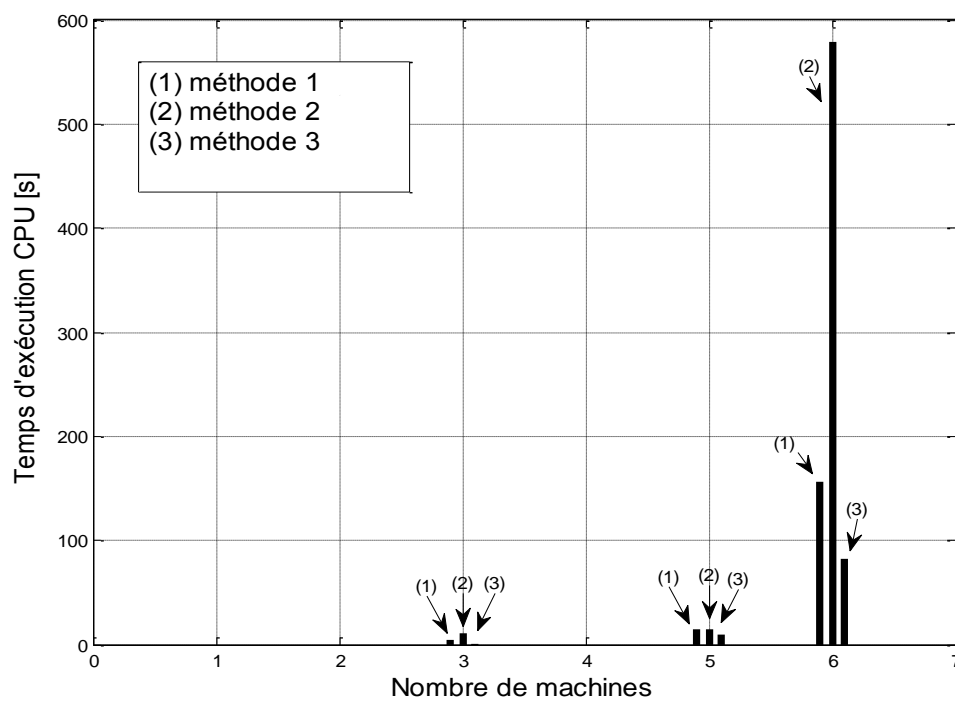
Figure II. 20 : Variation du temps d'exécution en fonction du nombre de machines
