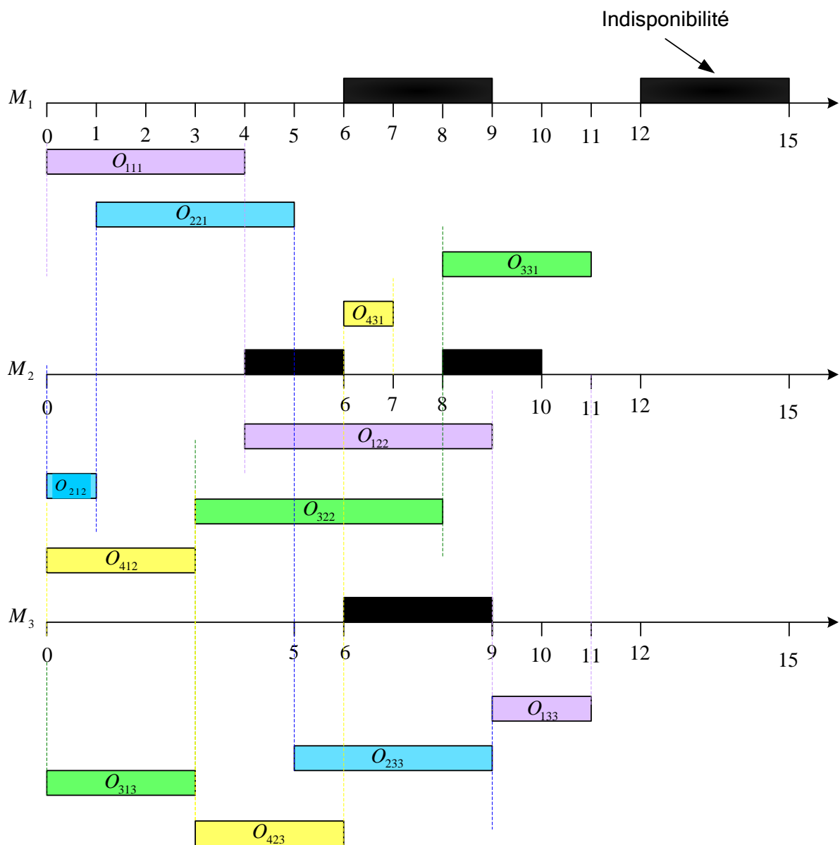
Figure III. 12 : Allocation des opérations aux machines suivant la règle 1 à l'instant t=0
