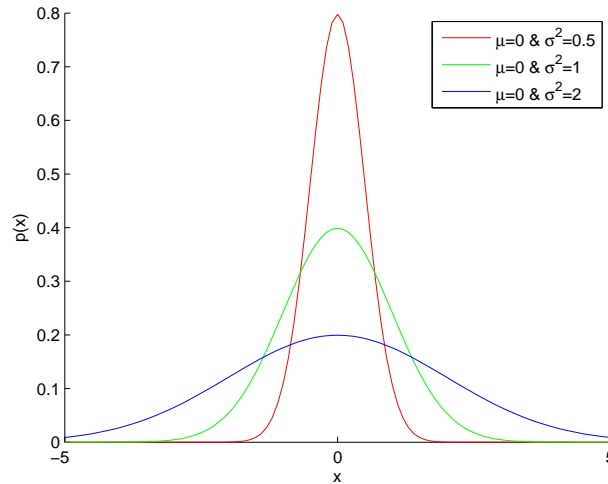
FIGURE 1.16 – Loi normale de moyenne nulle ( \mu = 0 ), pour différentes variances ( \sigma^2 \in [0.5, 1, 2] )
