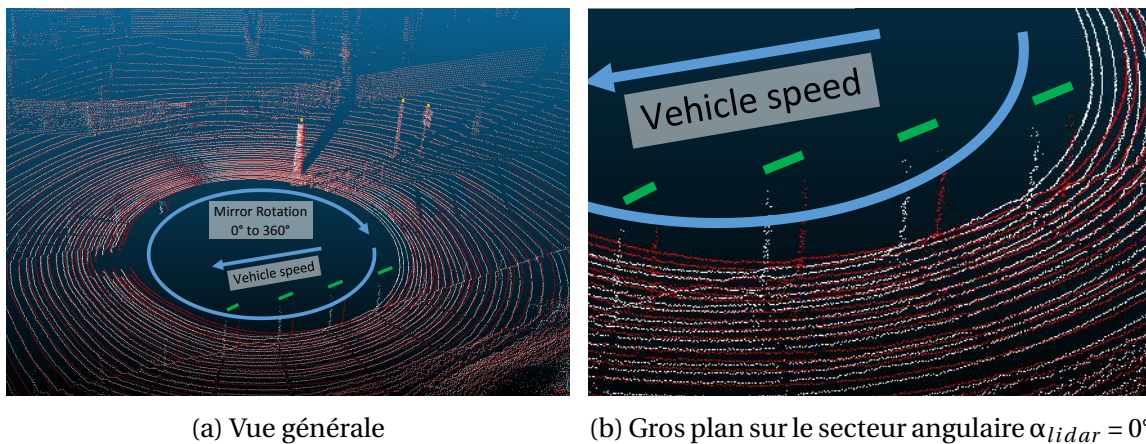
FIGURE B.4 – Déformation des scans LiDAR due à une translation du véhicule à une vitesse de 10m/s. Scan brut (blanc) et scan corrigé par l'odométrie (rouge) : les déformations sont faibles pour \alpha_{lidar} = 360^\circ , les objets sont confondus; alors que pour \alpha_{lidar} = 0^\circ les déformations sont d'environ 1m, les poteaux au premier plan sont décalés d'1m (lignes vertes).
