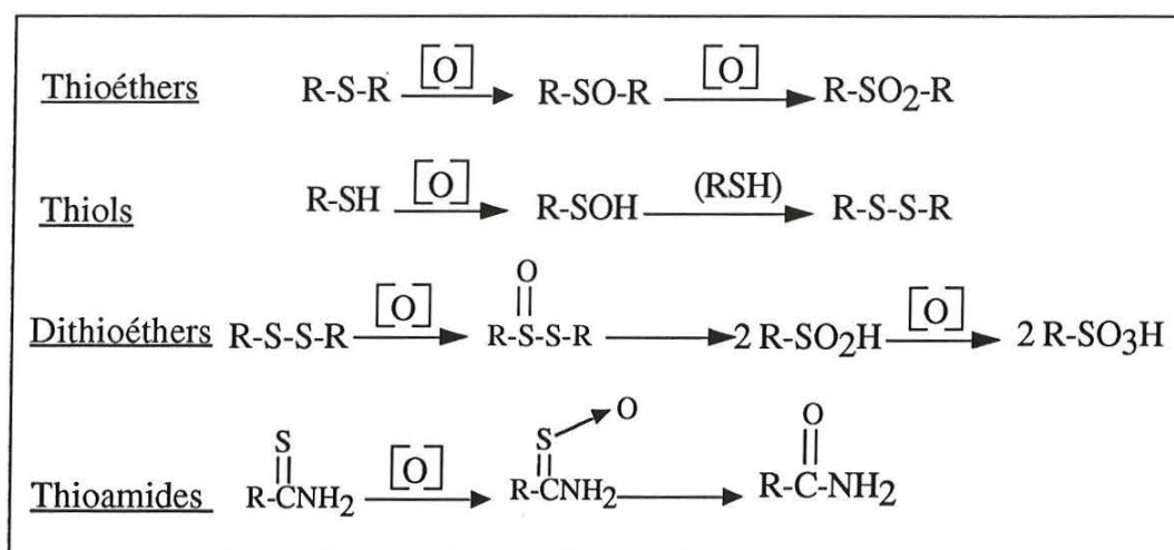
Figure 1-15 Quelques exemples d'oxydation métabolique de dérivés soufrés.
