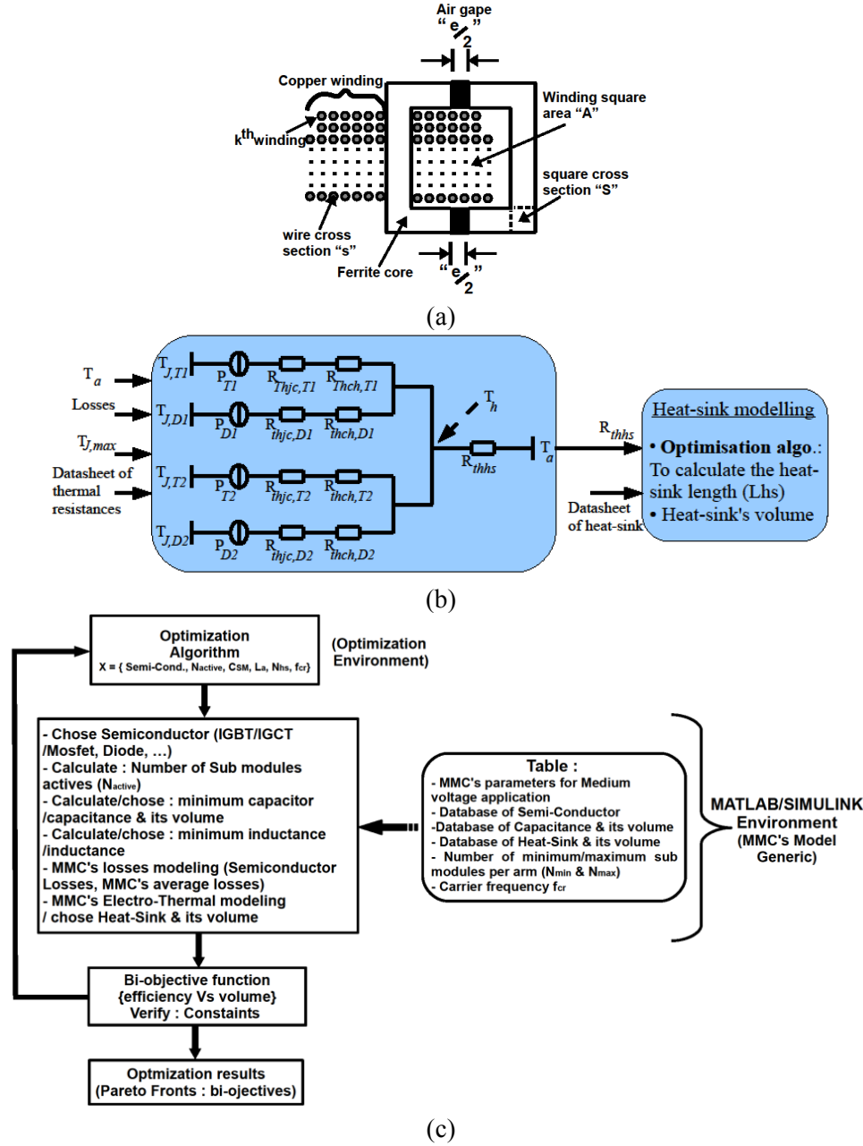
Fig. 2: Les outils de pré-dimensionnement de MMC
