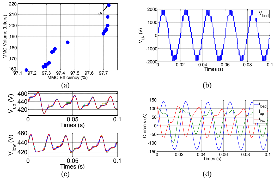
Fig. 3: Les résultats de simulation
