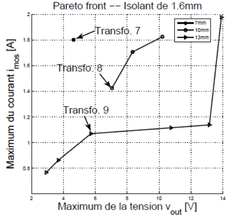
a. PCB Insulation layer 1.6 mm
