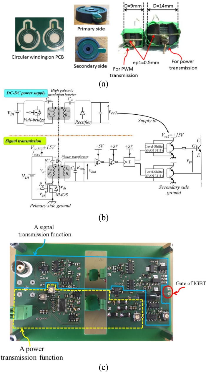
Fig. 8: Prototype des transformateurs et des fonctions étudiées
