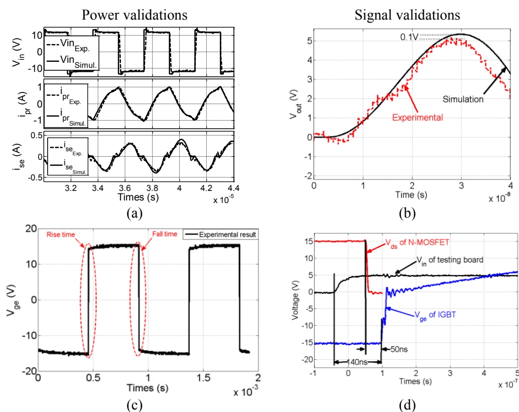
Fig. 9: Résultats expérimentaux d'un driver pour la distance d'isolante de 0.5mm
