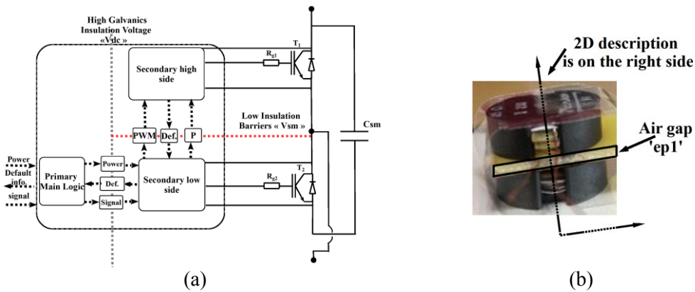
Fig. 4: Nouvelle architecture de commande rapprochées pour les deux IGBTs dans le SM-MMC et transformateur planaire.
