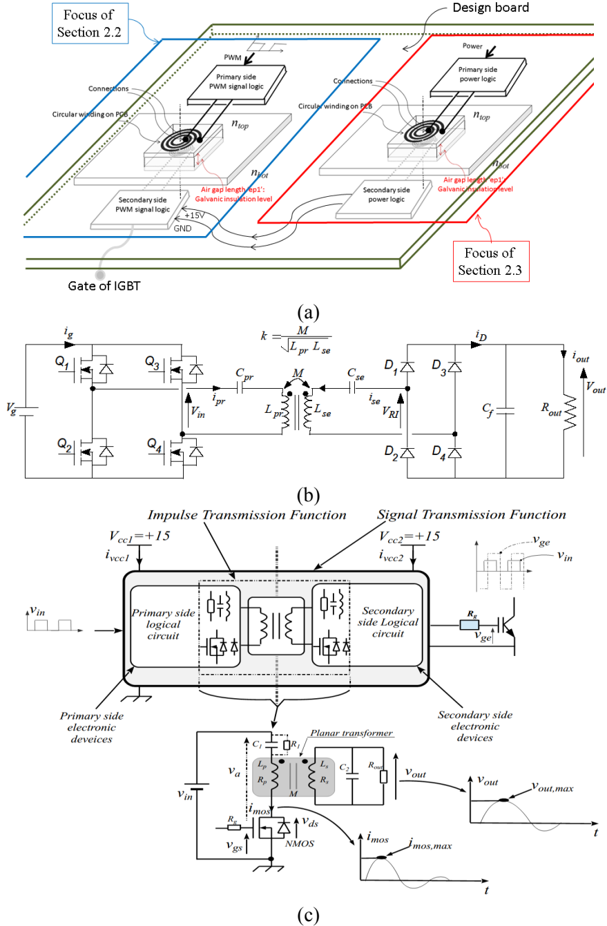
Fig. 5: Circuits électriques des fonctions de transmission puissance et de transmission d'ordre
