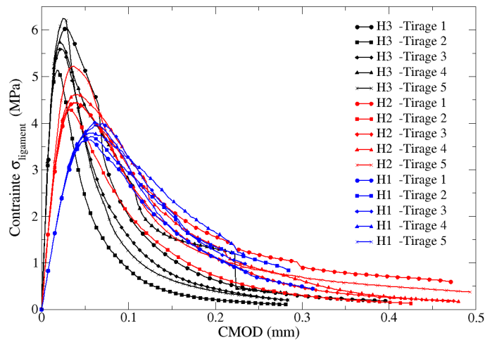
(b) Contraincte dans le ligament-CMOD
