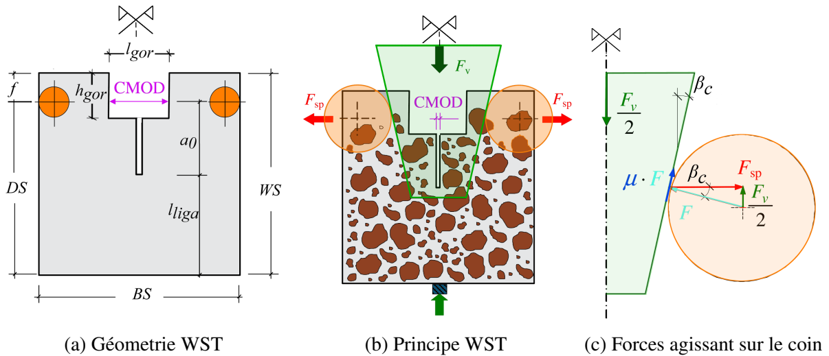
FIGURE 3.1 – L'essai Wedge Splitting : principes, géométrie et conditions limites
