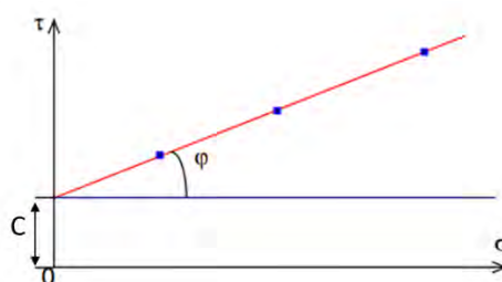
Figure A9.2 : Courbe intrinsèque obtenue après 3 essais effectués à 3 contraintes \sigma appliquées
