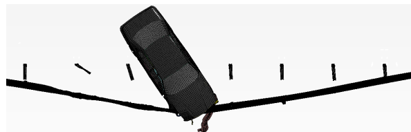
Figure A- 16 Échec de la réorientation du véhicule : H et E diminuent considérablement
