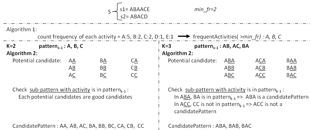
FIGURE 4.4 – Illustration de la création des patterns candidats. S est l'ensemble des séquences, min\_fr est le seuil de fréquence, K est la longueur des patterns candidats à créer, pattern_{k-1} sont les patterns fréquents de longueur k - 1 .
