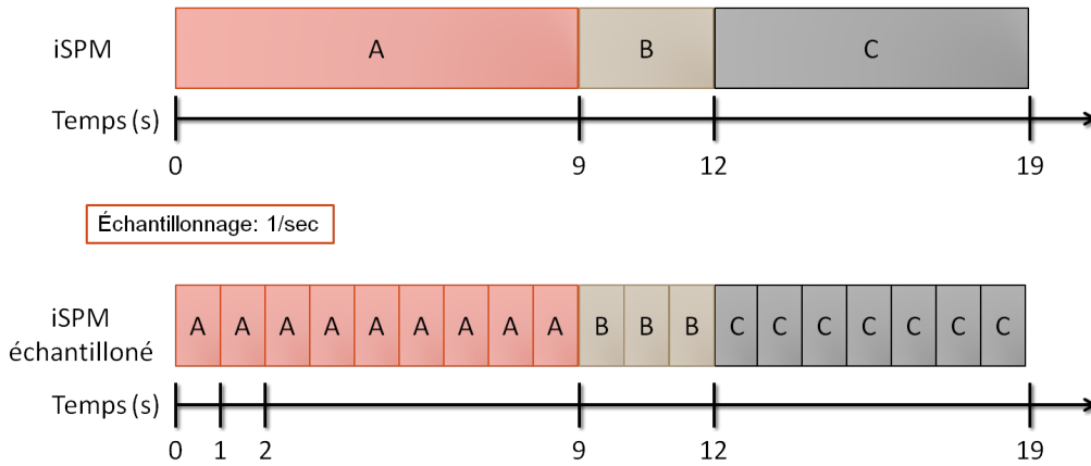
FIGURE 3.3 – Échantillonnage d’un iSPM continu (en haut) pour obtenir un iSPM discret (en bas). Avant échantillonnage, les activités ont des durées différentes, 9 secondes pour A , 3 secondes pour B et 7 secondes pour C . Après échantillonnage, toutes les activités ont la même durée, cependant A est répété 9 fois, B 3 fois et C 7 fois.
