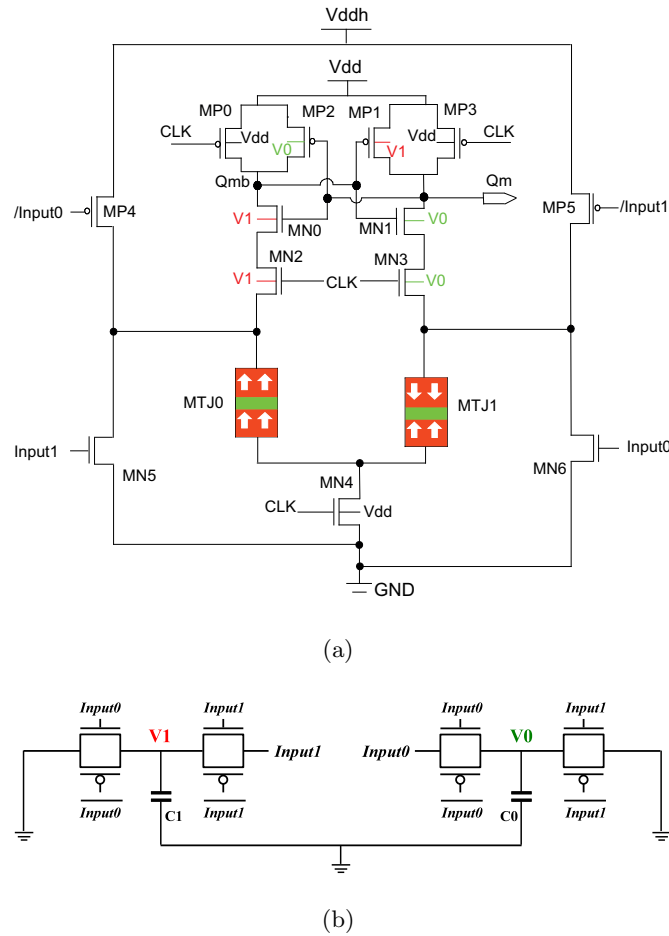
Figure B.16: (a) Amplificateur de détection de pré-charge avec polarisation du substrat asymétrique dynamique (b) Les circuits RC génèrent les tensions de polarisation du substrat pour les transistors dans PCSA.
