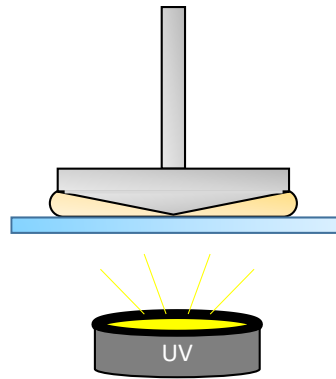
Figure 141 : système d'exposition aux UV in situ dans le rhéomètre.
