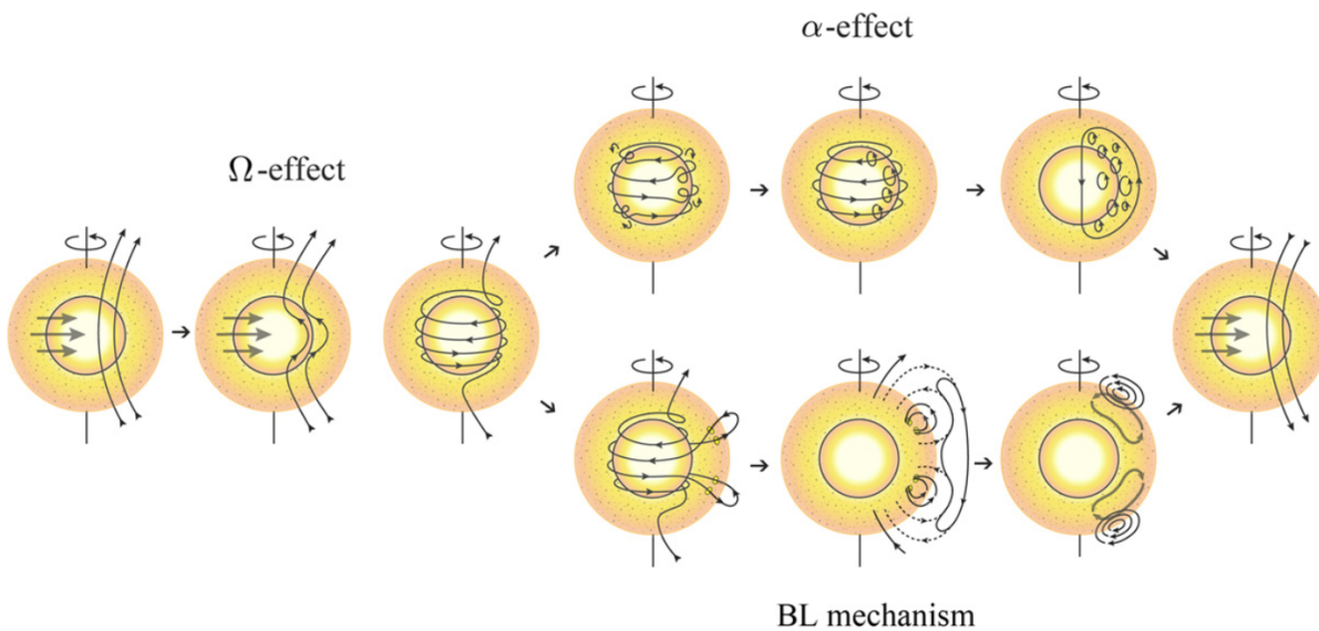
Figure 2.3 – Illustration des processus principaux en jeu dans les modèles de dynamo solaire. L'effet \Omega (à gauche) décrit la transformation d'un champ magnétique initialement poloïdal en un champ toroïdal, à cause de la rotation différentielle solaire. Le passage du champ toroïdal au champ poloïdal est ensuite décrit soit par l'effet \alpha (en haut) ou par l'effet Babcock-Leighton (BL, en bas) (figure tirée de Sanchez et al., 2014).
