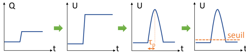
Figure 6.11 – Chaîne électronique.
