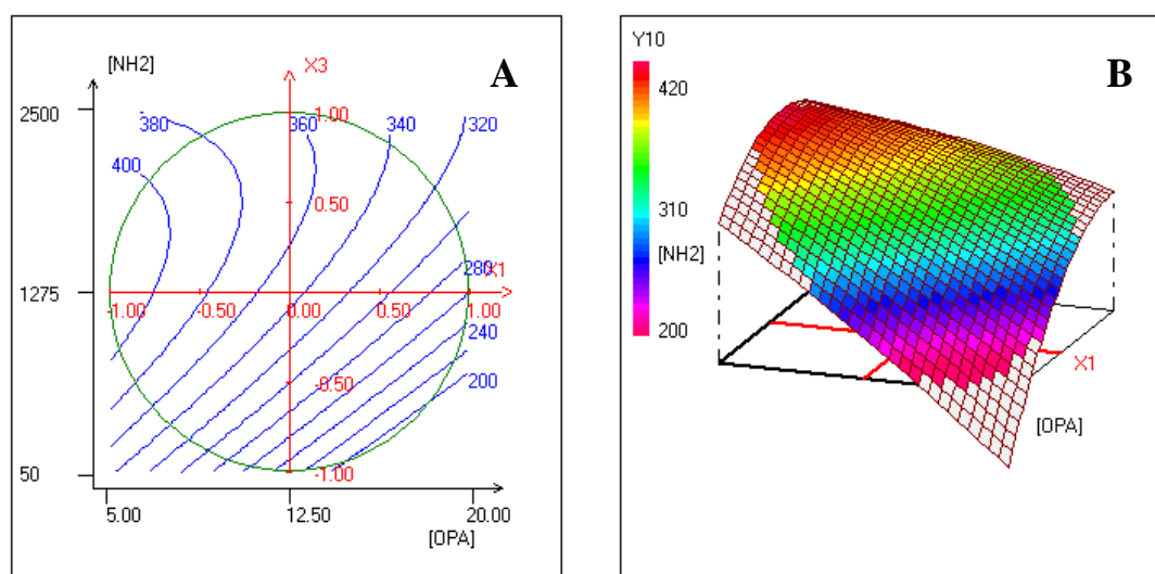
Figure 52 : Courbes de niveau (A) et de surface de réponse (B) montrant la variation de la réponse Y_{10} (Intensité de fluorescence) en fonction de [OPA] ( X_1 ) et [AE] ( X_3 ). Le pourcentage de méthanol dans le solvant réactionnel a été fixé à 50%.
