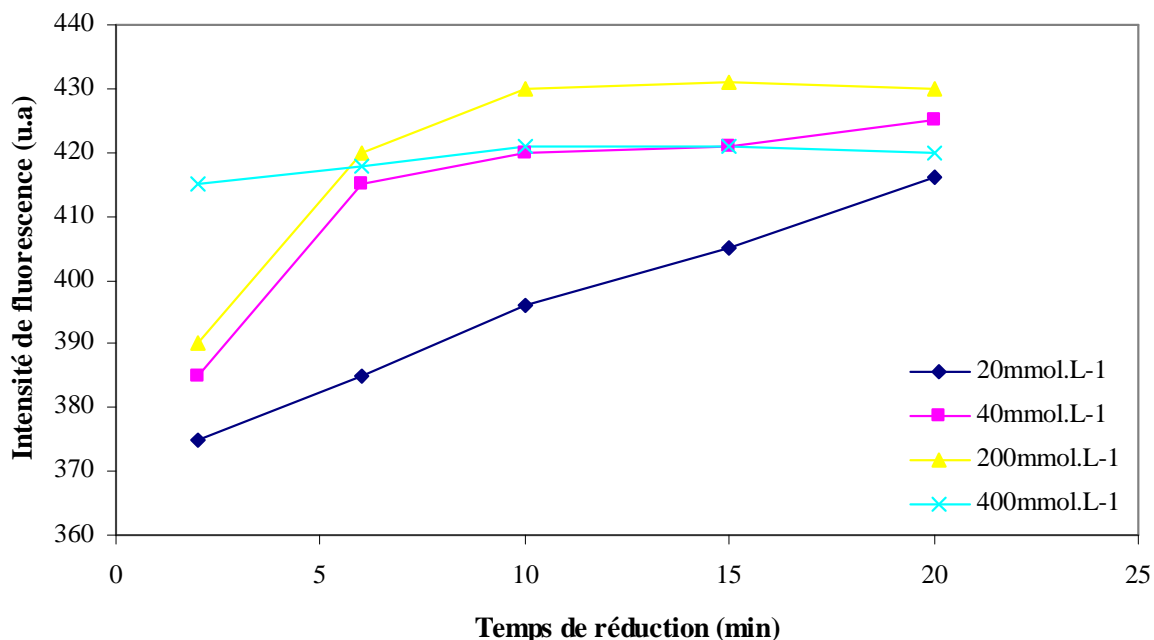
Figure 57 : Cinétiques de réduction de CSSC à différents concentrations de TBP à \lambda_{em} = 445 \text{ nm} ( \lambda_{ex} = 335 \text{ nm} ), \text{pH} = 9,5 , [\text{OPA}] = 50 \mu\text{mol.L}^{-1} , [\text{AE}] = 13,5 \text{ mmol.L}^{-1} , \text{MeOH} = 43\%
