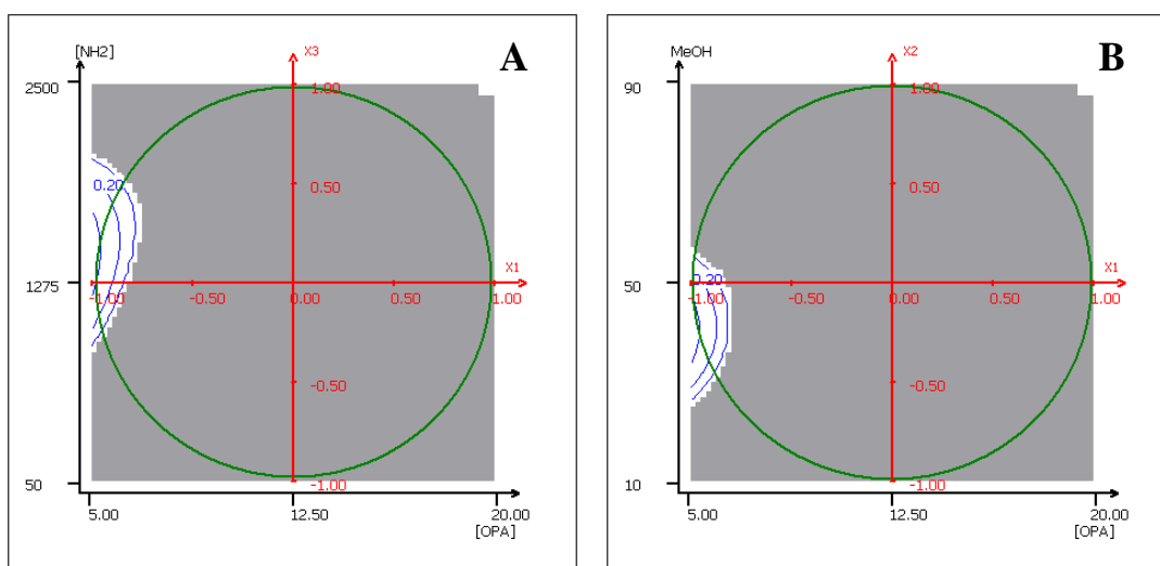
Figure 54 : Courbes d'isoresponses de la fonction de désirabilité. (A) concentration en OPA, concentration en aminoéthanol avec 43% MeOH (facteur fixe). (B) Concentration en OPA et %MeOH avec [AE] de 14 \text{ mmol.L}^{-1} (facteur fixe).
