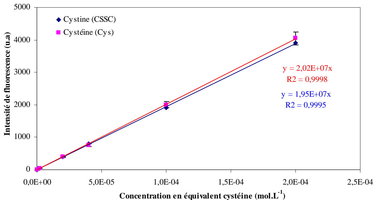
Figure 58: Corrélation entre l'intensité de fluorescence et les concentrations en équivalents de cystéine à \lambda_{em}= 445 \text{ nm} ( \lambda_{ex}= 335 \text{ nm} ), \text{pH}= 9,5 , [\text{OPA}]= 50 \mu\text{mol.L}^{-1} , [\text{AE}]= 13,5 \text{ mmol.L}^{-1} , \text{MeOH}= 43\% , [\text{TBP}]= 200 \text{ mmol.L}^{-1}
