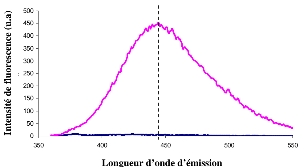
Figure 30 : Réponse spectrale du dérivé fluorescent à \lambda_{\text{em}} = 445\text{nm} ( \lambda_{\text{exc}} = 335\text{nm} ).
