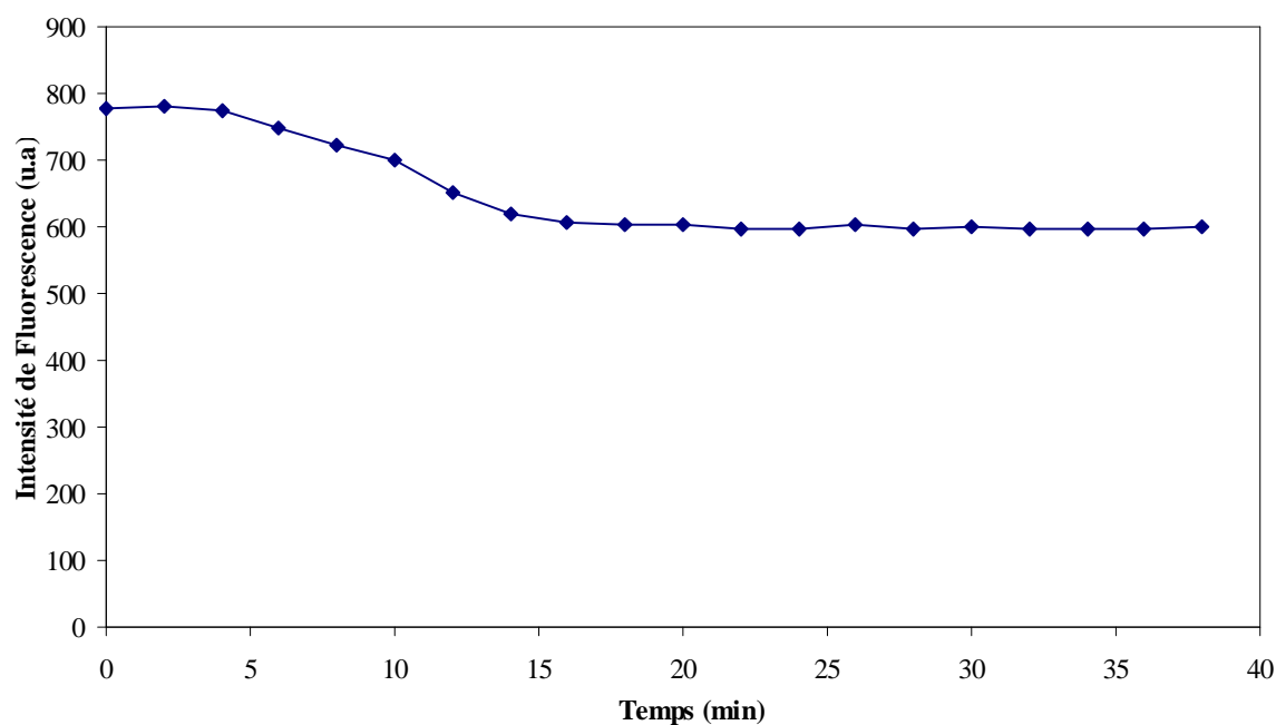
Figure 39: Stabilité de fluorescence du dérivé ammonium formé à \lambda_{em} = 485\text{nm} . [\text{OPA}] = 3 \text{ mmol.L}^{-1} , [\text{NAC}] = 3 \text{ mmol.L}^{-1} , pH : 10,8
