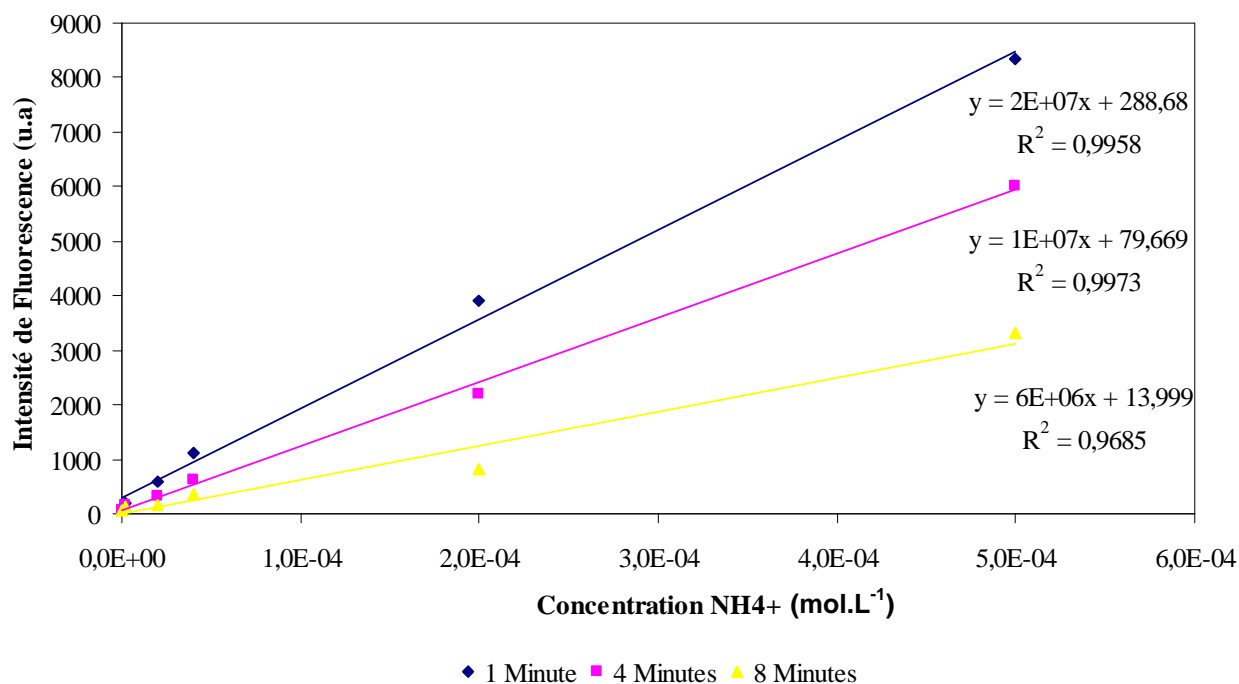
Figure 42: Evolution des droits d'étalonnage du dérivé ammonium à \lambda_{\text{em}} = 455 \text{ nm} ( \lambda_{\text{em}} = 335 \text{ nm} ) [\text{OPA}] = 3 \text{ mmol.L}^{-1} , [\text{NAC}] = 3 \text{ mmol.L}^{-1} , \text{pH} = 10,8
