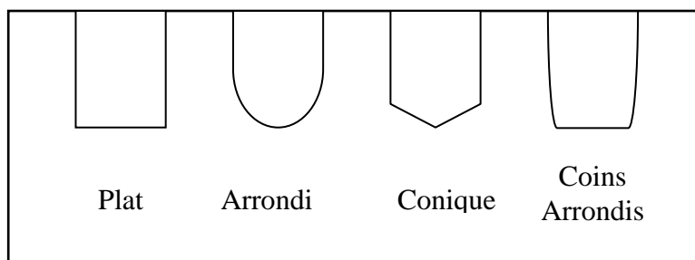
Figure 17 : Les quatre géométries de fonds de puits disponibles sur les microplaques: fonds plats (fond F), fonds ronds (fond U), fonds coniques (fond V), fonds à coins arrondis avec un fond plat (fond C).
