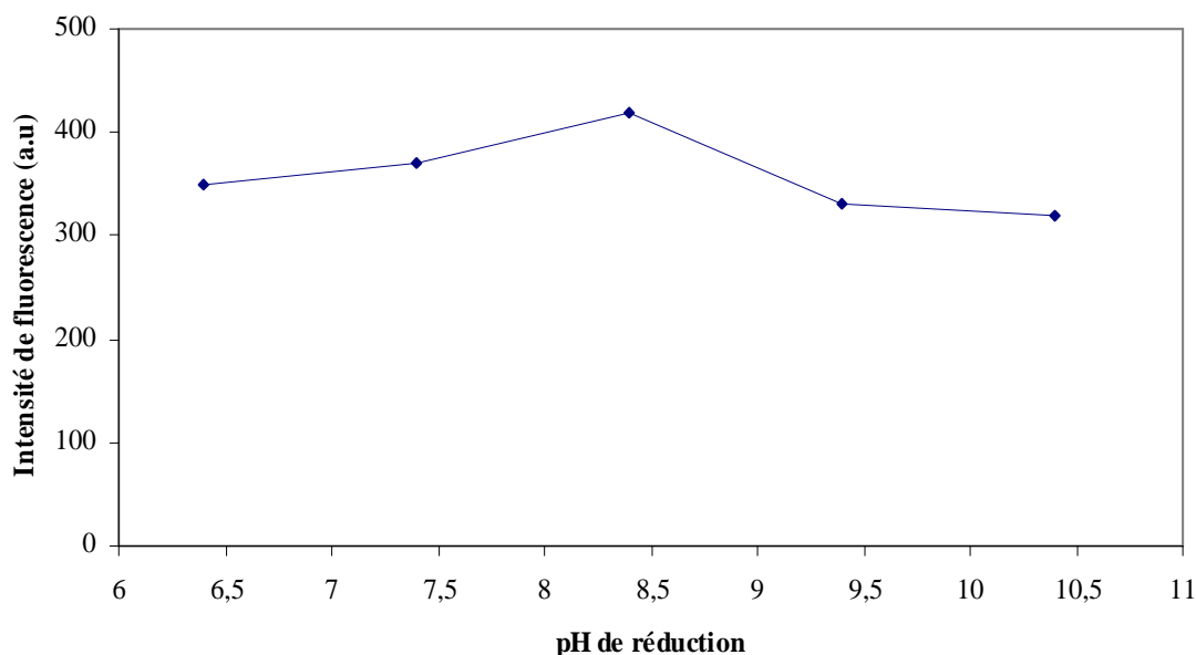
Figure 56: Influence du pH sur dans l'étape de réduction à : \lambda_{em} = 445 \text{ nm} ( \lambda_{ex} = 335 \text{ nm} ), [\text{OPA}] = 50 \mu\text{mol.L}^{-1} , [\text{AE}] = 13,5 \mu\text{mol.L}^{-1} , \text{MeOH} = 43\%
