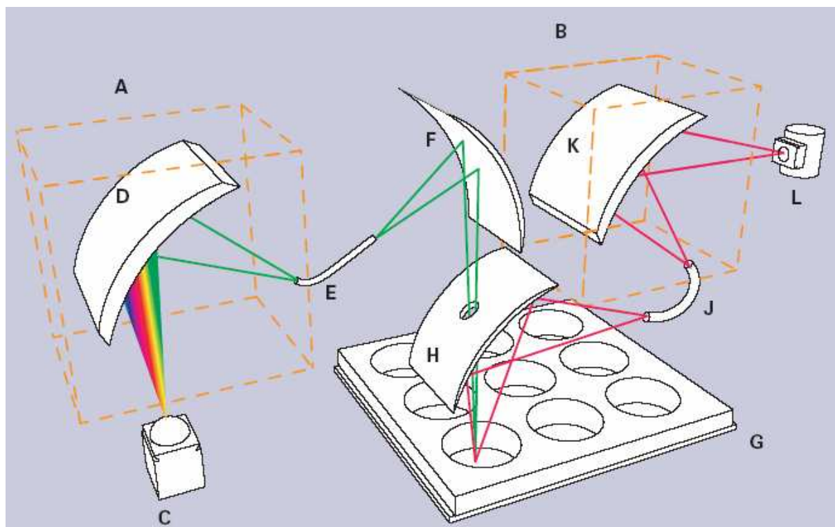
Figure 18: Fonctionnement d'un lecteur microplaque (d'après la brochure Spectramax, Geminis XS Molecular Devices).
