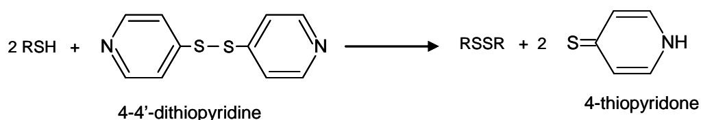
Figure 10 : Formation de la thiopyridone en présence de composés thiols et de dithiopyridine
