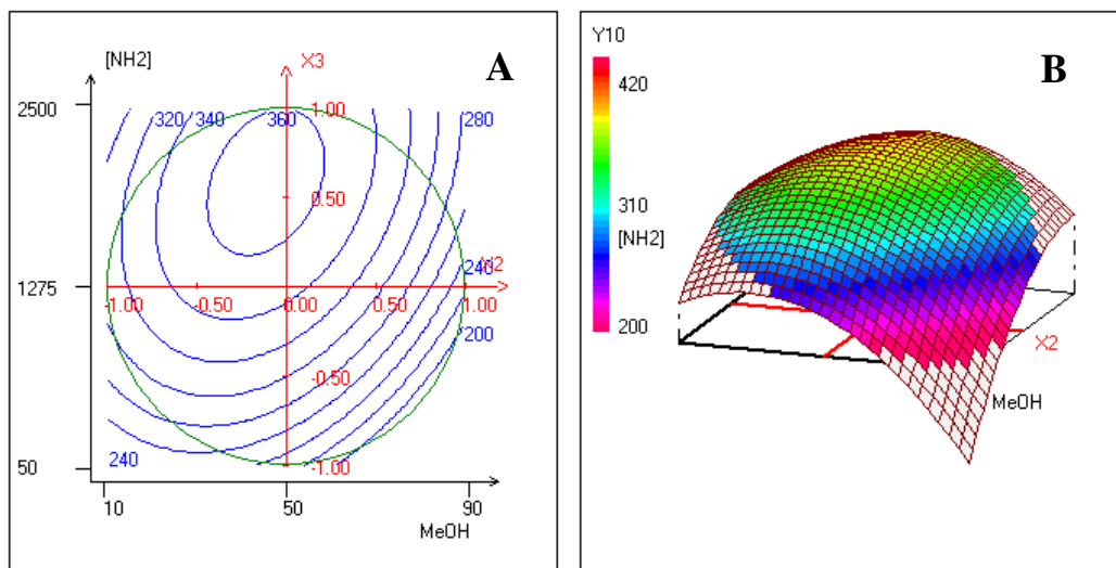
Figure 53 : Courbes de niveau (A) et de surface de réponse (B) montrant la variation de la réponse Y_{10} (Intensité de fluorescence) en fonction de [%MeOH] ( X_2 ) et [AE] ( X_3 ). La concentration en OPA a été fixée à 125 \mu\text{mol.L}^{-1} .
