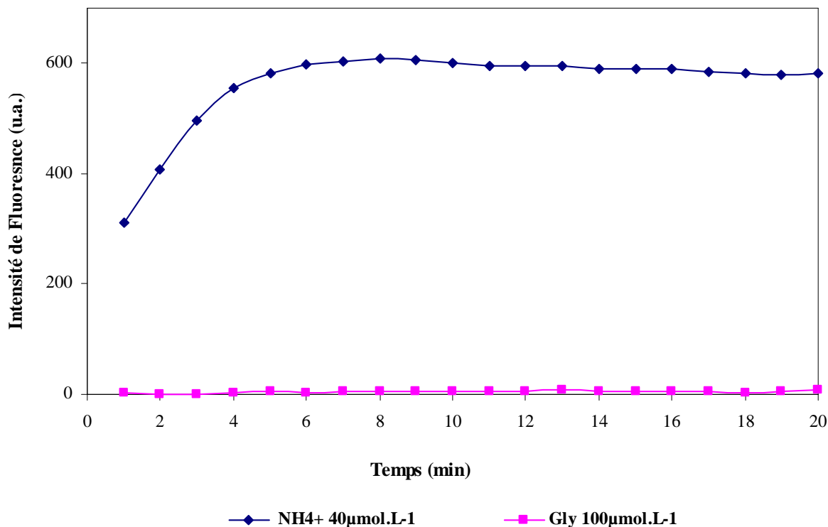
Figure 38: Cinétique de stabilité du dérivé isoindole en présence de \text{NH}_4^+ et de glycine à \lambda_{em} = 485 nm ( \lambda_{ex} = 415 nm)
