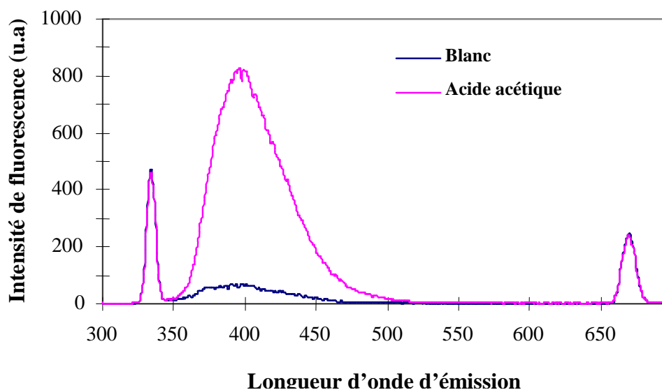
Figure 34 : Réponse spectrale du dérivé fluorescent à \lambda_{em} = 395 nm ( \lambda_{exc} = 335 nm).
