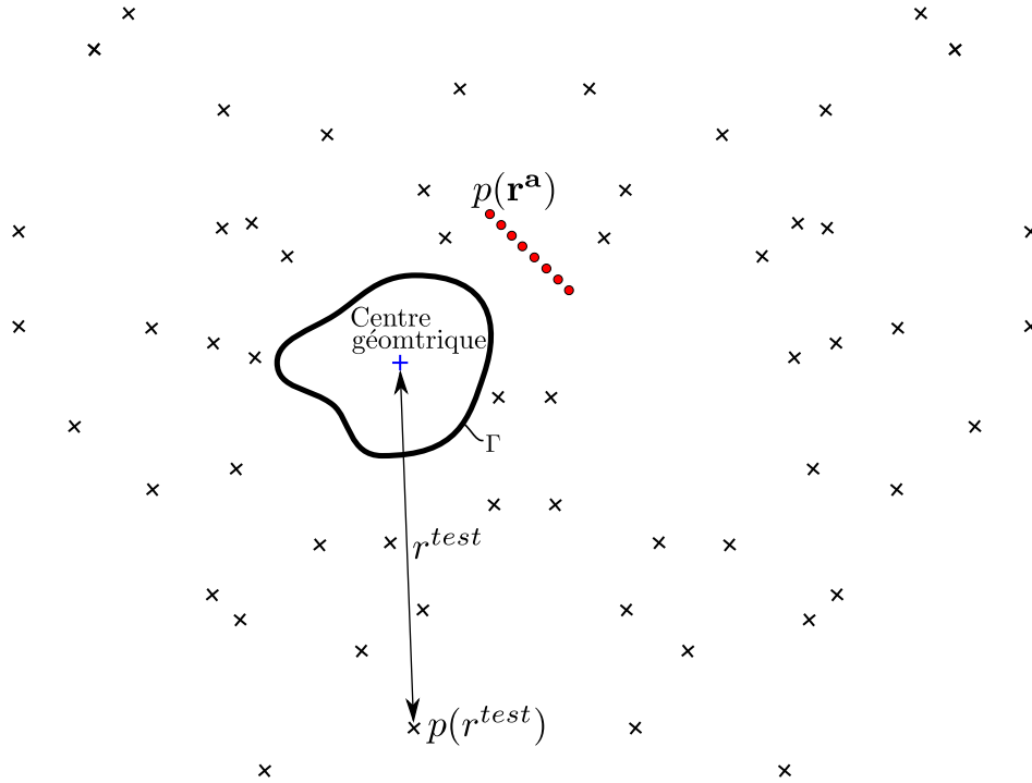
Figure 4.3 – Schéma de la configuration géométrique utilisée permettant de forcer un a priori de rayonnement omnidirectionnel autour de l'objet d'intérêt. Les points rouges, la croix bleue et les croix noires représentent successivement la position des microphones de l'antenne réelle, le centre géométrique de l'objet et les microphones virtuels.
