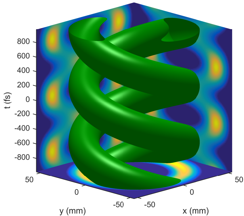
FIGURE 130 – Représentation dans le domaine (x, y, t) de l’intensité du champ électrique d’un faisceau LS du second ordre. Isosurface à 20 % du maximum et projection sur les plans (x, t) , (y, t) et (x, y)
