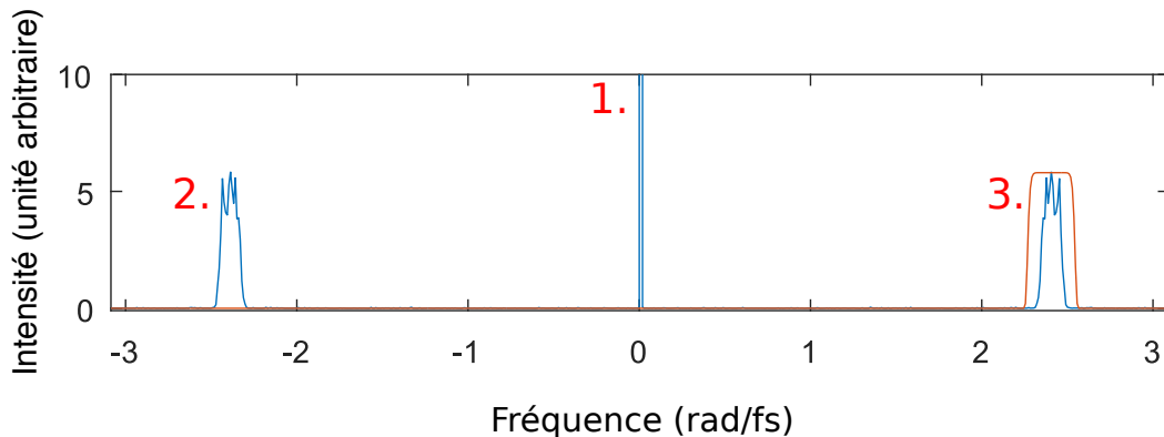
FIGURE 32 – Intensité de la transformée de Fourier suivant le délai du signal TERMITES de la figure 28
