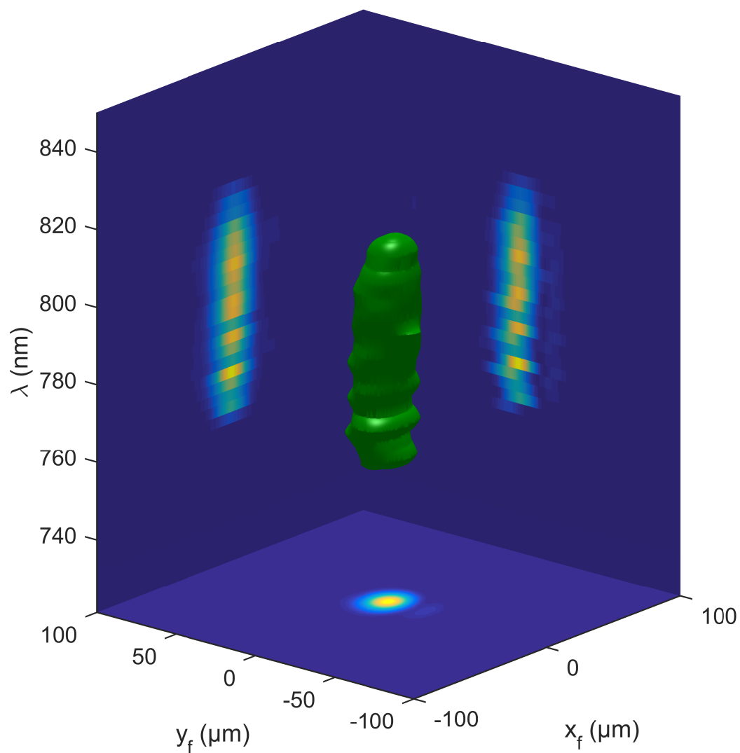
FIGURE 82 – Représentation de la tache focale résolue spectralement à l'aide d'une iso-surface à 5% de l'intensité maximale et de projections sur les plans (x_f, \lambda) , (y_f, \lambda) et (x_f, y_f)
