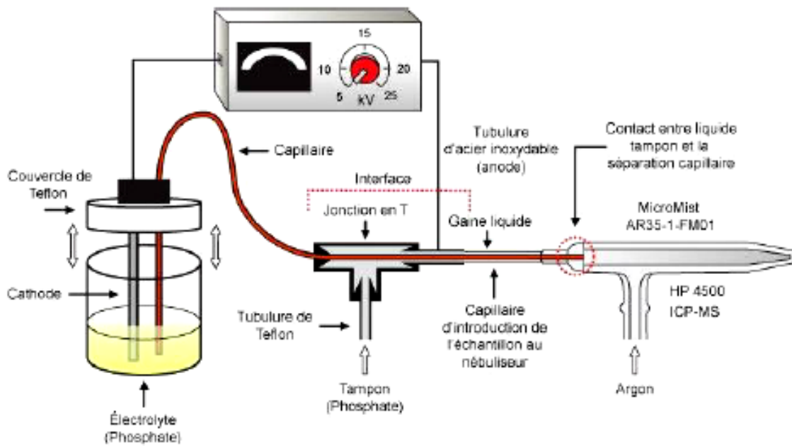
Fig 57 : Principe de l'électrophorèse capillaire
