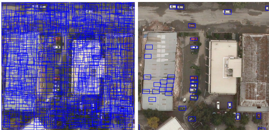
FIGURE 4.5 – À gauche hypothèses de détections provenant de plusieurs modèles avant la fusion. A droite hypothèses filtrés par la Non Maximum Suppression (NMS) : plusieurs orientations de véhicules sont conservées (y compris les faux positifs sur le toit).
