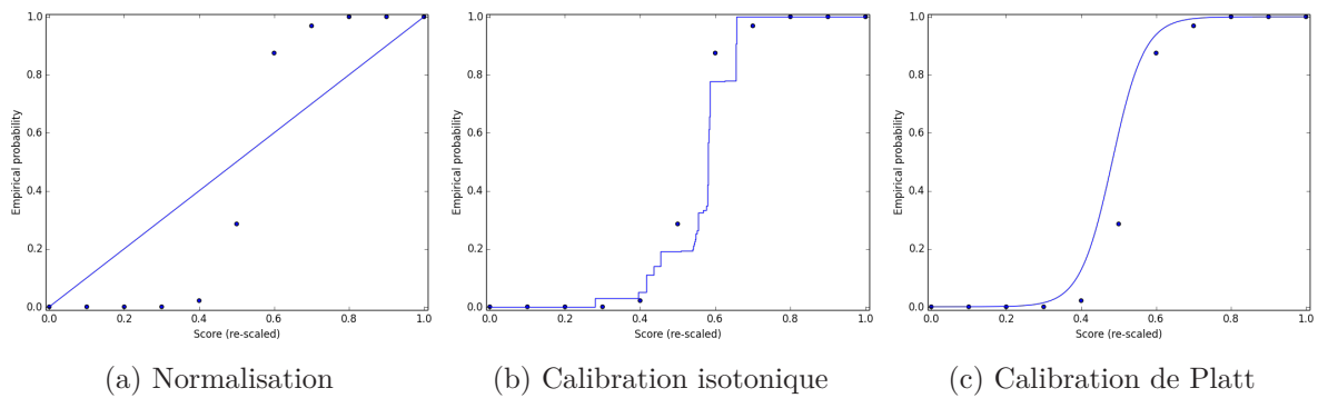
FIGURE 4.6 – Illustration des différentes méthodes de calibration des classificateurs. Pour chacune des figures les points sont les scores bruts d’une SVM. La courbe quant à elle représente la nouvelle répartition des scores après calibration.
