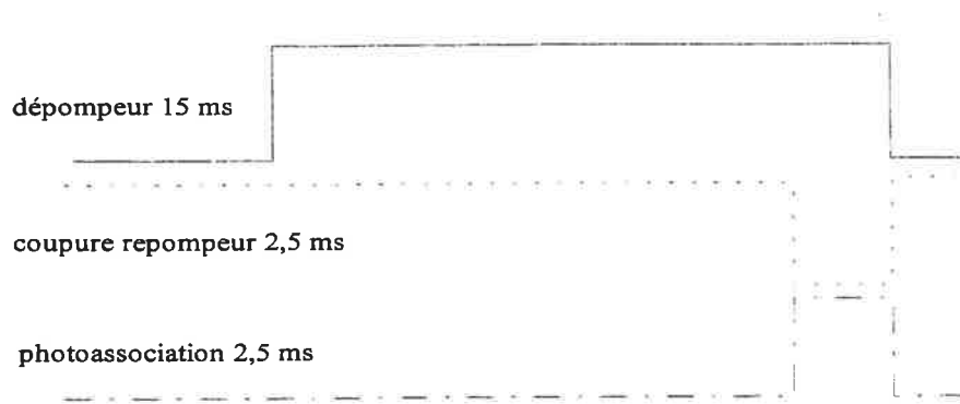
FIG. 1.6: Schéma de pompage des atomes vers F=3 .
