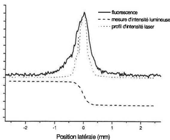
FIG. 1.20: Comparaison de l'extension spatiale du piège magnéto-optique (trait plein), et du waist du laser de photoassociation (pointillés). Ce dernier est déterminé par la méthode suivante : on obstrue partiellement la tâche laser par une lame de rasoir montée sur vis micrométrique. Celle-ci est déplacée, et on enregistre l'intensité laser après la lame en fonction de la position de la lame (tirets). Le profil d'intensité du laser est la dérivée du signal mesuré en fonction de la position de la lame.
