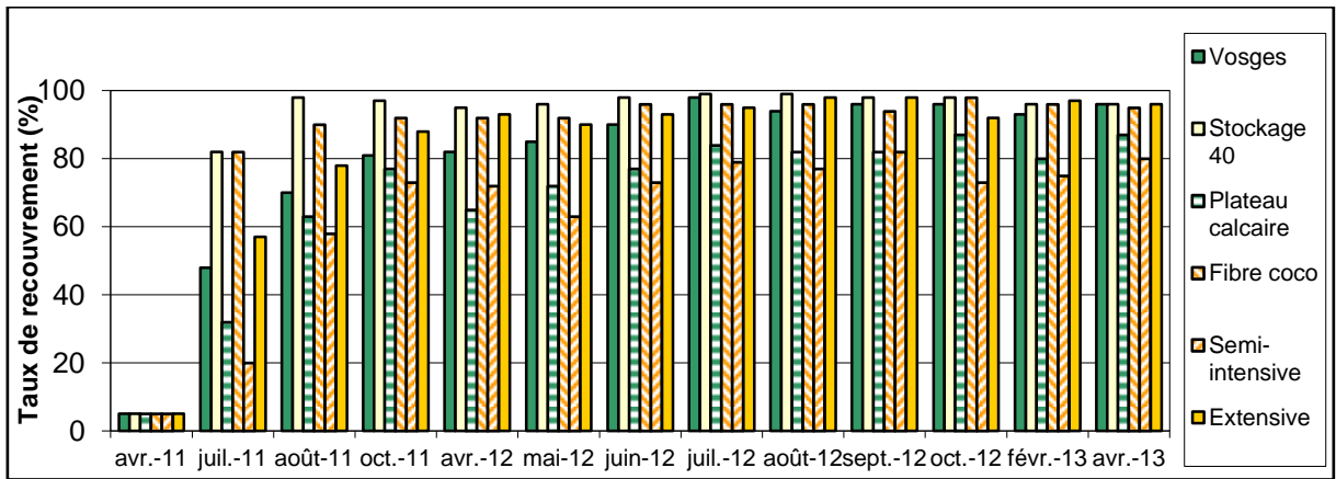
Figure 41 - Evolution du pourcentage de recouvrement par la végétation des différentes toitures d'avril 2011 à avril 2013
